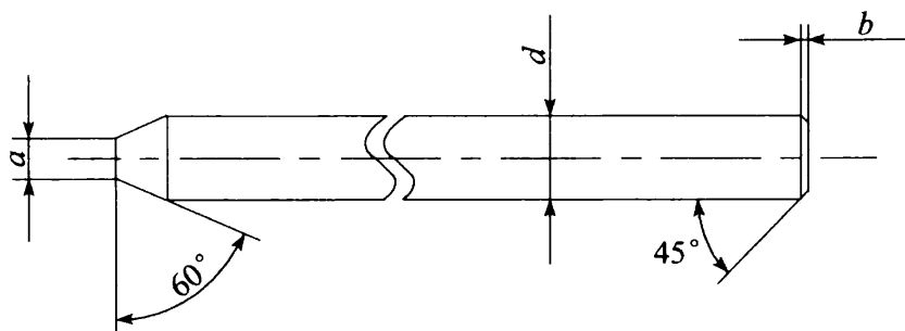
图 3.2.8-1 无螺纹结构(一头平一头尖)示意图
