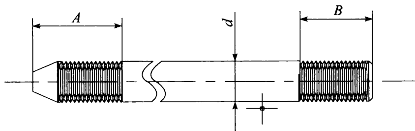
图 3.2.8-2 有螺纹结构(一端带尖)示意图
