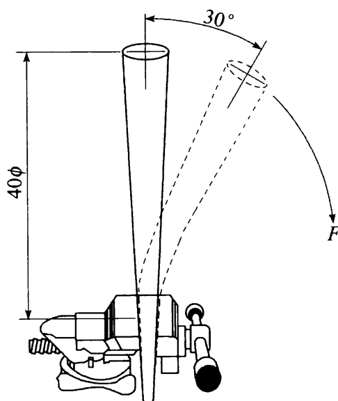
图 4.0.4 电铸铜接地棒(线)弯折性能试验示意图
