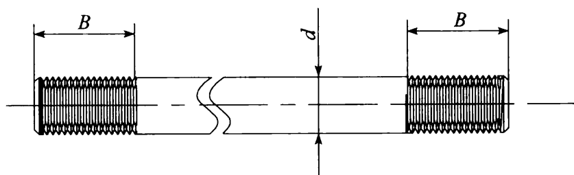
图 3.2.8-3 有螺纹结构(两端平)示意图
