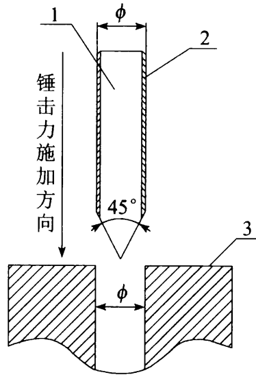
图 4.0.5 电铸铜接地棒(线)结合性试验示意图
