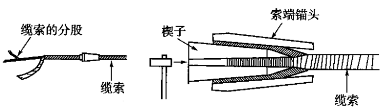
图 3.2.2-1 缆索的分股和楔子锚固
