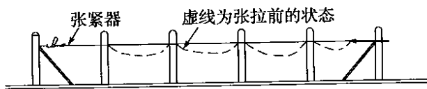
图 3.2.2-2 临时张拉缆索
