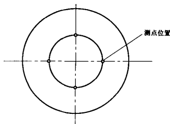
图 4 圆形风口测点布置
