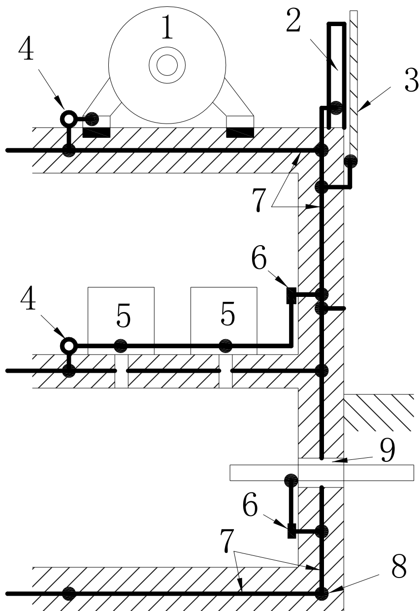
图 D.0.4-1 钢筋混凝土建筑物等电位连接位置
