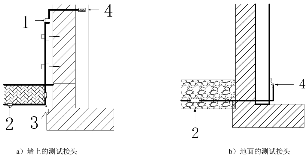
图 D.0.1-1 在建筑物地面处连接板（测试点）的安装
