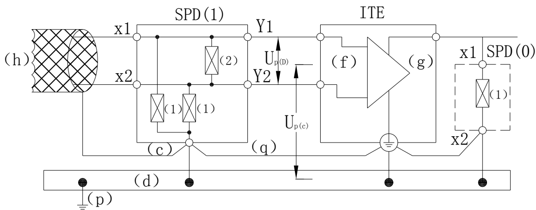
图 D.0.6-1 电子设备的信号（f）和低压配电输入（9）的共模电压和差模电压的防护措施示例
