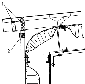
图 5.3.3 檐口构造
