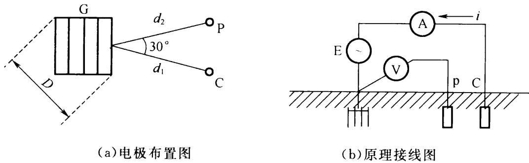
图 A.0.4 三角法的原理接线图
