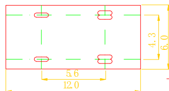
260t 汽车平面尺寸
