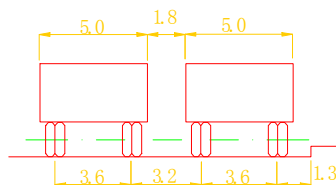
110t 汽车横向布置
