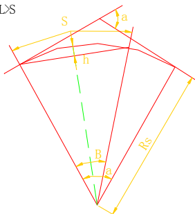
附图 4.1 不设回旋曲线时横净距计算图
