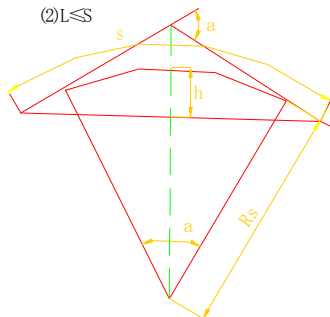
附图 4.1 不设回旋曲线时横净距计算图
