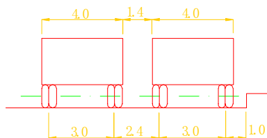
80t 汽车横向布置
