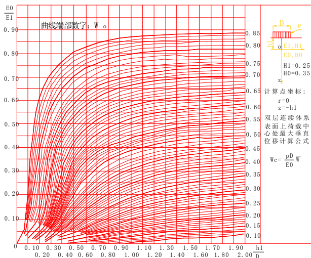
图 4.3.7 弹性层状体系精确图解
