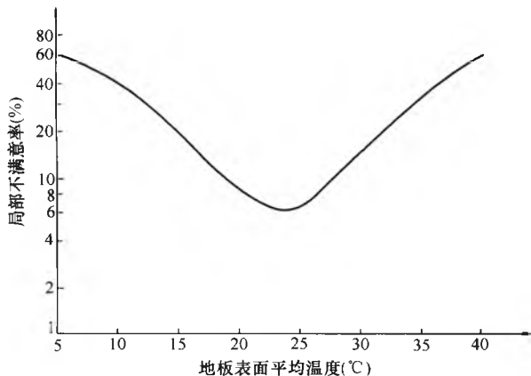
图 F.0.3 地板表面温度引起的局部不满意率
