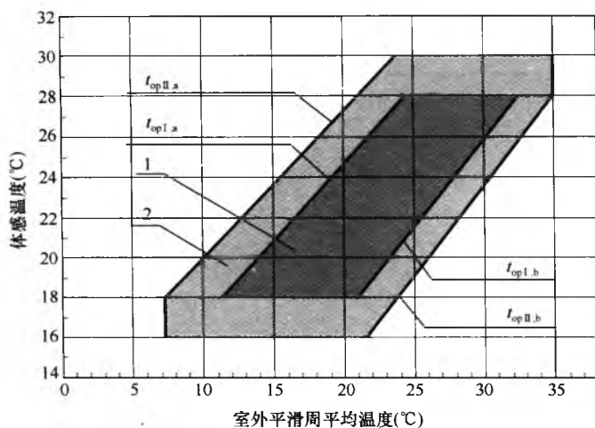
图 5.2.4-2 夏热冬冷、夏热冬暖、温和地区非人工冷热源 热湿环境体感温度范围
