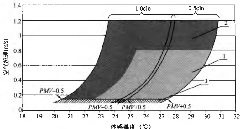
图 4.2.5-2 抵消空气温度上升需要的空气流速
