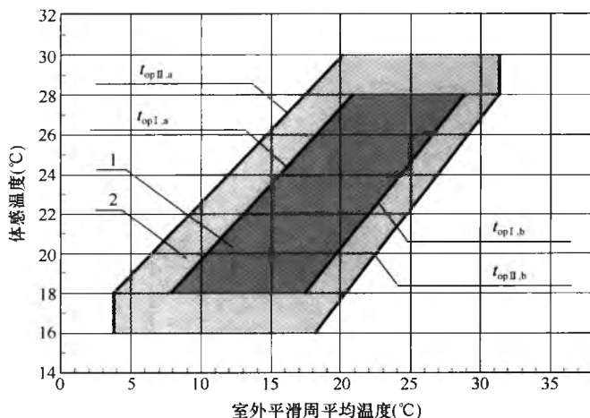
图 5.2.4-1 严寒及寒冷地区非人工冷热源热湿 环境体感温度范围
