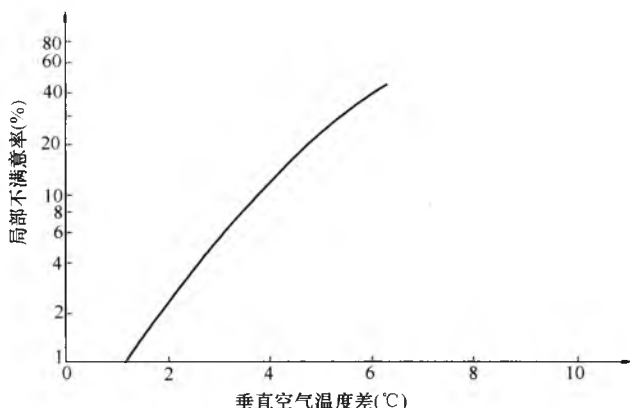
图 F.0.2 由垂直空气温度差引起的局部不满意率
