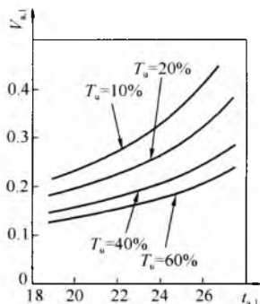
图 1 空气温度、空气流速和空气紊流强度关系图
