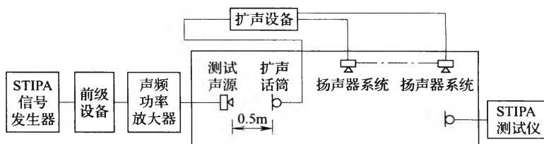
图 1 STIPA 声输入法测量方框图
