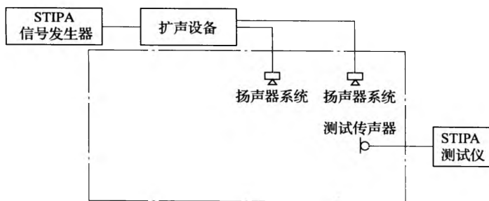
图 6.4.3 STIPA 测量原理框图
