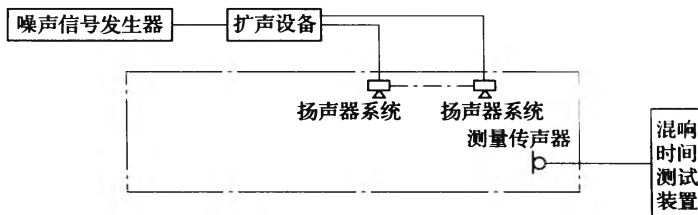
图 6.4.1 声衰变时间测量原理框图
