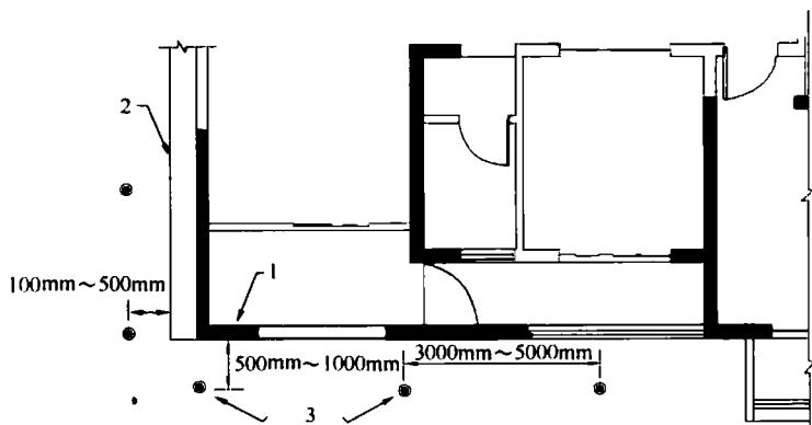
图 4.2.2 常见白蚁监测装置安装示意图
