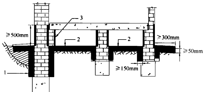
(b) 架空层结构房屋
