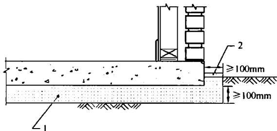
图 6.2.1 底层非架空楼板结构砂粒屏障设置
