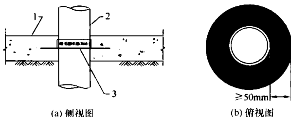
图 3.1.6 管道防蚁圈的安装
