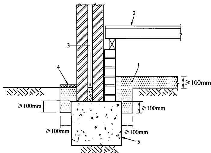
图 6.2.2 底层架空楼板结构砂粒屏障设置
