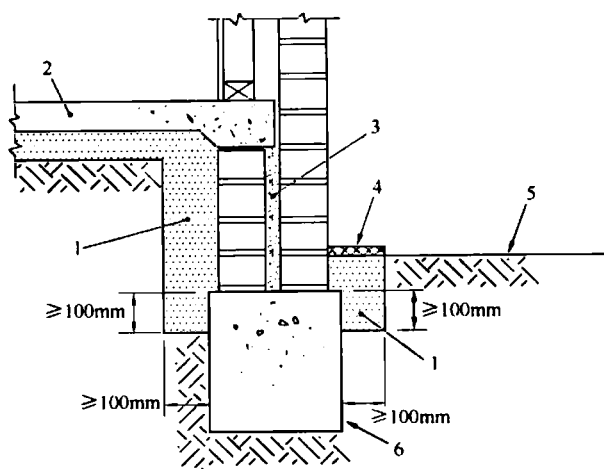
图 6.2.3 房屋周围砂粒屏障设置
