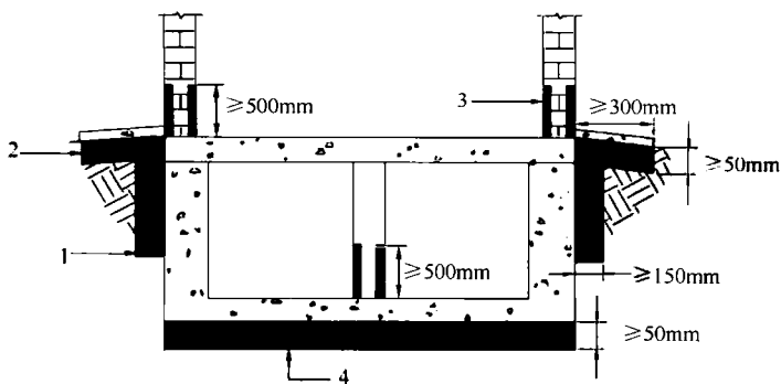
(c) 地下室结构房屋
