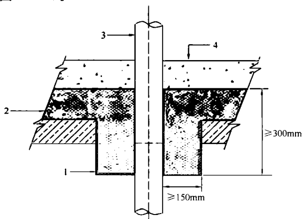
图 5.2.4 入户管道入口处药物土壤屏障设置
