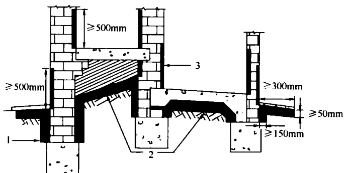
(a) 非架空层结构房屋
