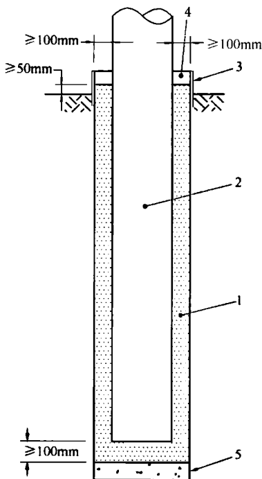
图 6.2.8 柱或支杆的砂粒屏障设置
