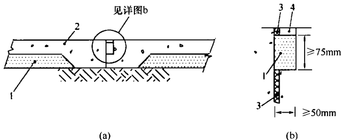
图 6.2.7 混凝土地坪沉降缝或伸缩缝砂粒屏障设置
