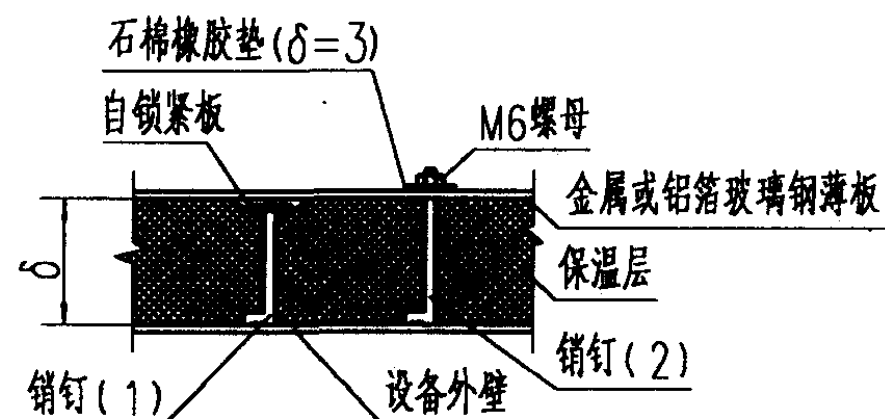
保温断面
