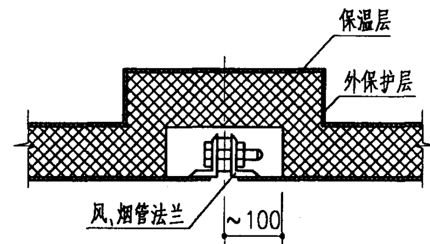
法兰保温
