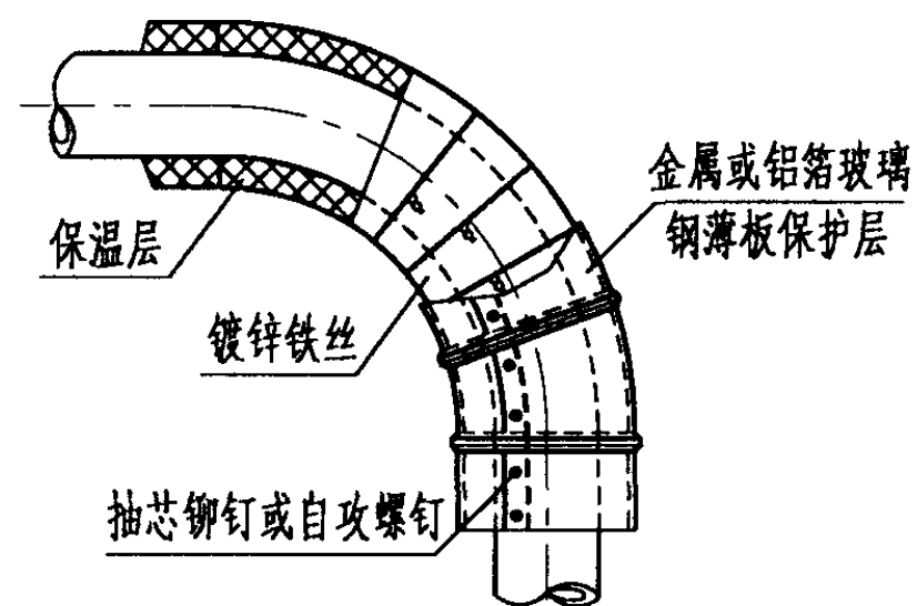
弯头(1)
