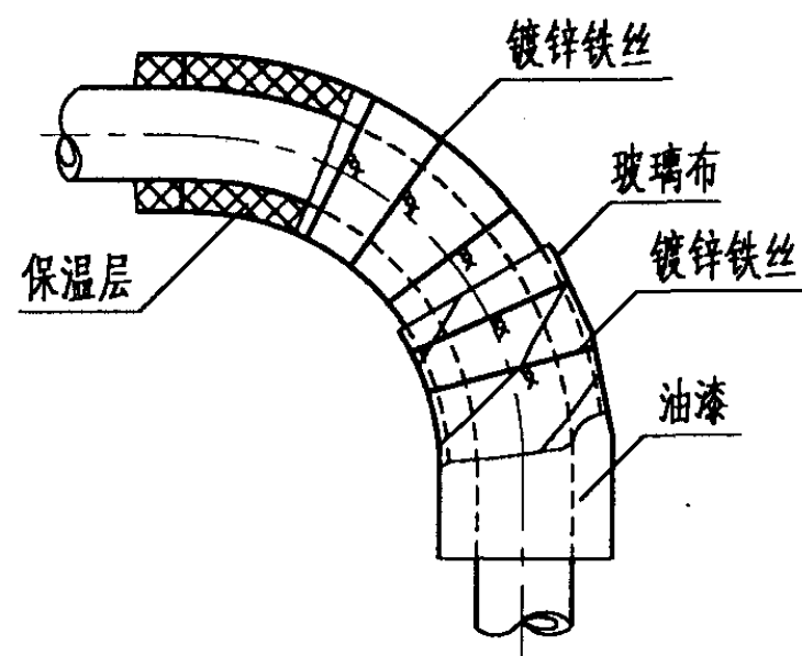
弯头(2)
