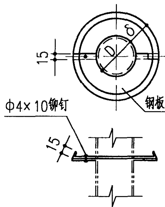
环形挂板
