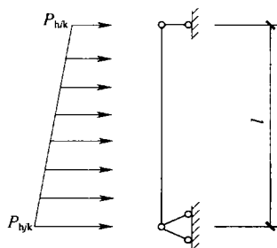
图 6.2.5 水平联梁间砌体计算简图
