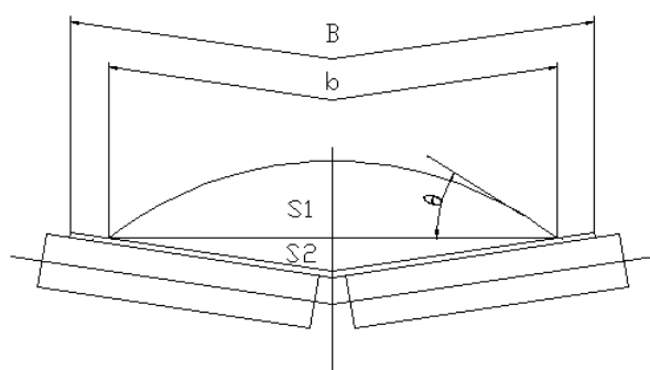
图 3.1.3-2 二托辊输送带上物料的横截面
