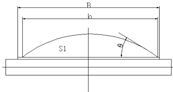
图 3.1.3-3 单托辊输送带上物料的横截面
