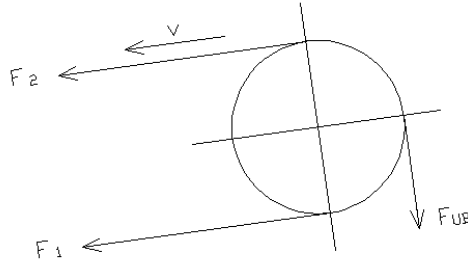
图 5.1.1-4 制动工况总阻力为负值的张力
