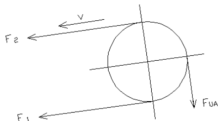
图 5.1.1-2 启动工况阻力为负值的张力
