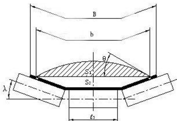
图 3.1.3-1 三托辊输送带上物料的横截面
