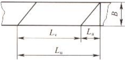
图 B.0.1 输送带硫化接头的长度
