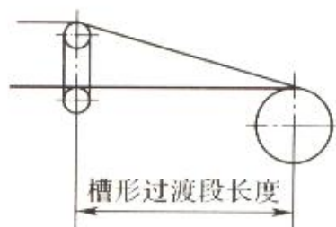
图 11.4.1-1 滚筒顶面位于槽形托辊组槽底面时， 槽形过渡段长度示意图
