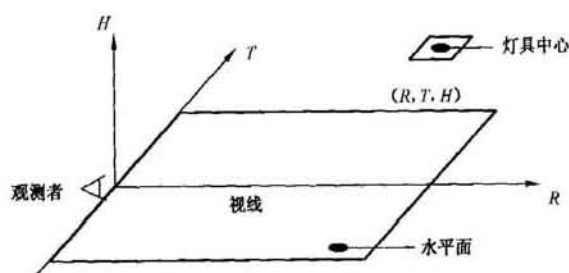
图 A.1 以观察者位置为原点的位置指数坐标系(R, T, H),对灯具中心生成 H/R 和 T/R 的比值
