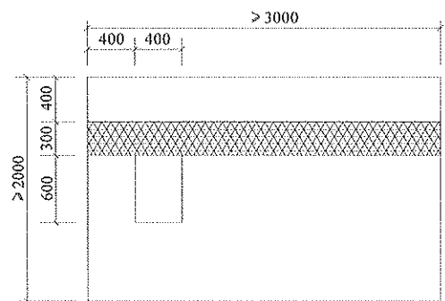
图 A.2.1-2 带防火隔离带试验墙板 (mm)
