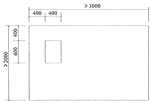
图 A.2.1-1 试验墙板 (mm)
