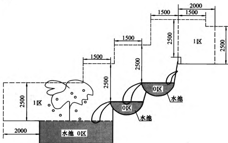
图 C. 0.2 喷水池区域划分
