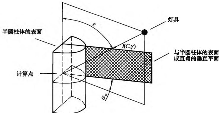
图 B. 0. 1 计算半柱面照度时所用的角
