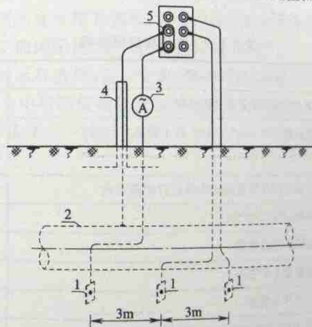
图 A.3.2 交流电流密度测量接线图
