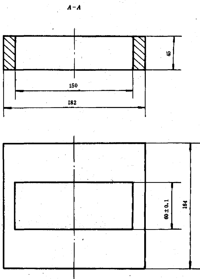
图 A3 模套
