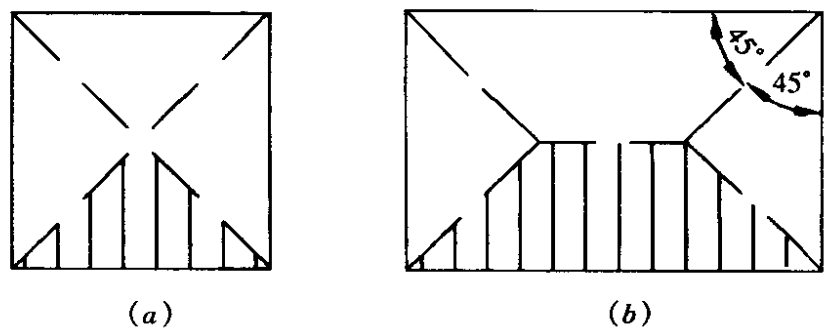
图 5.4.7 板面荷载向肋的传递 (a) 方板；(b) 矩形板
