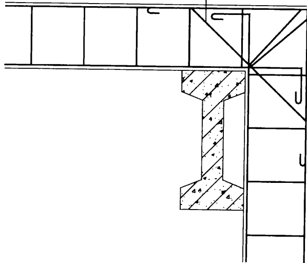
图 3 厂房转角处增设水平斜筋示意图
