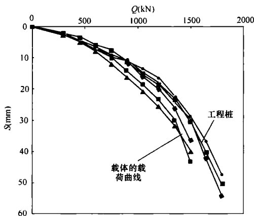
图 2 载体和载体桩曲线对比
