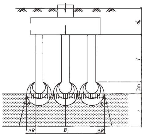
图 4.2.5 软弱下卧层计算示意
