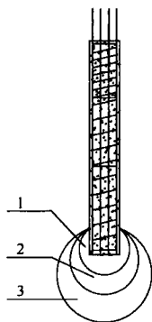
图4.3.1 抗拔载体桩构造
