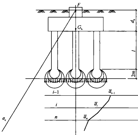
图 4.4.4 沉降计算示意
