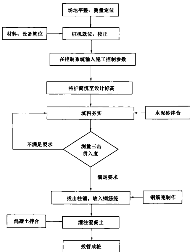
图 6.0.4 载体桩施工工艺
