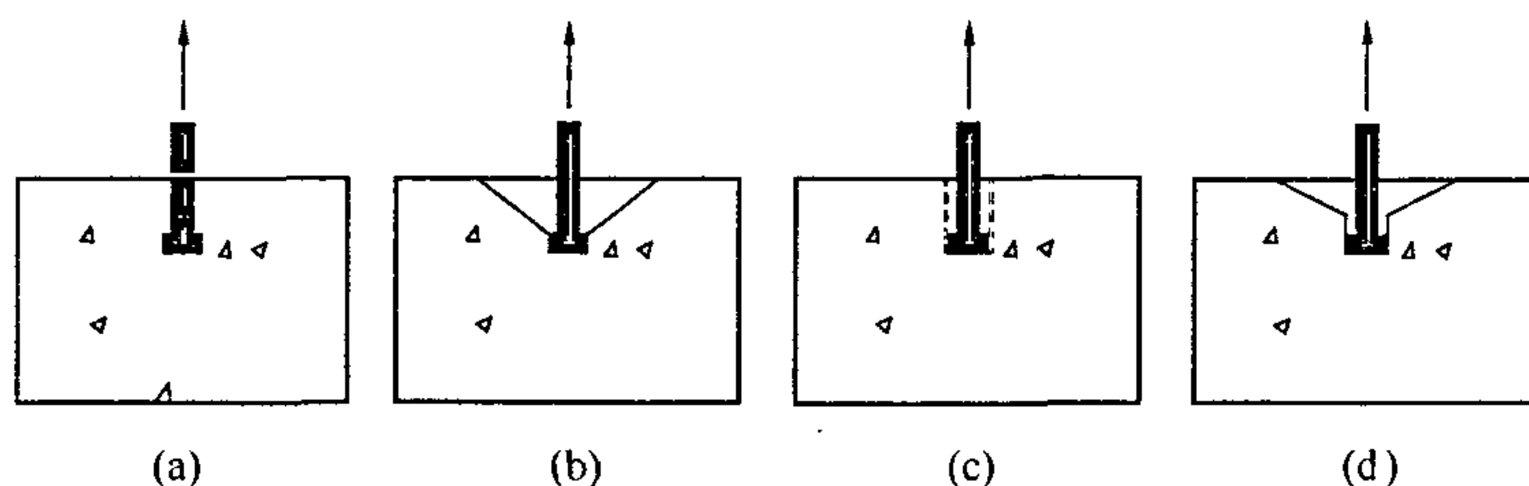
图 1 后锚固法破坏体破坏形式
