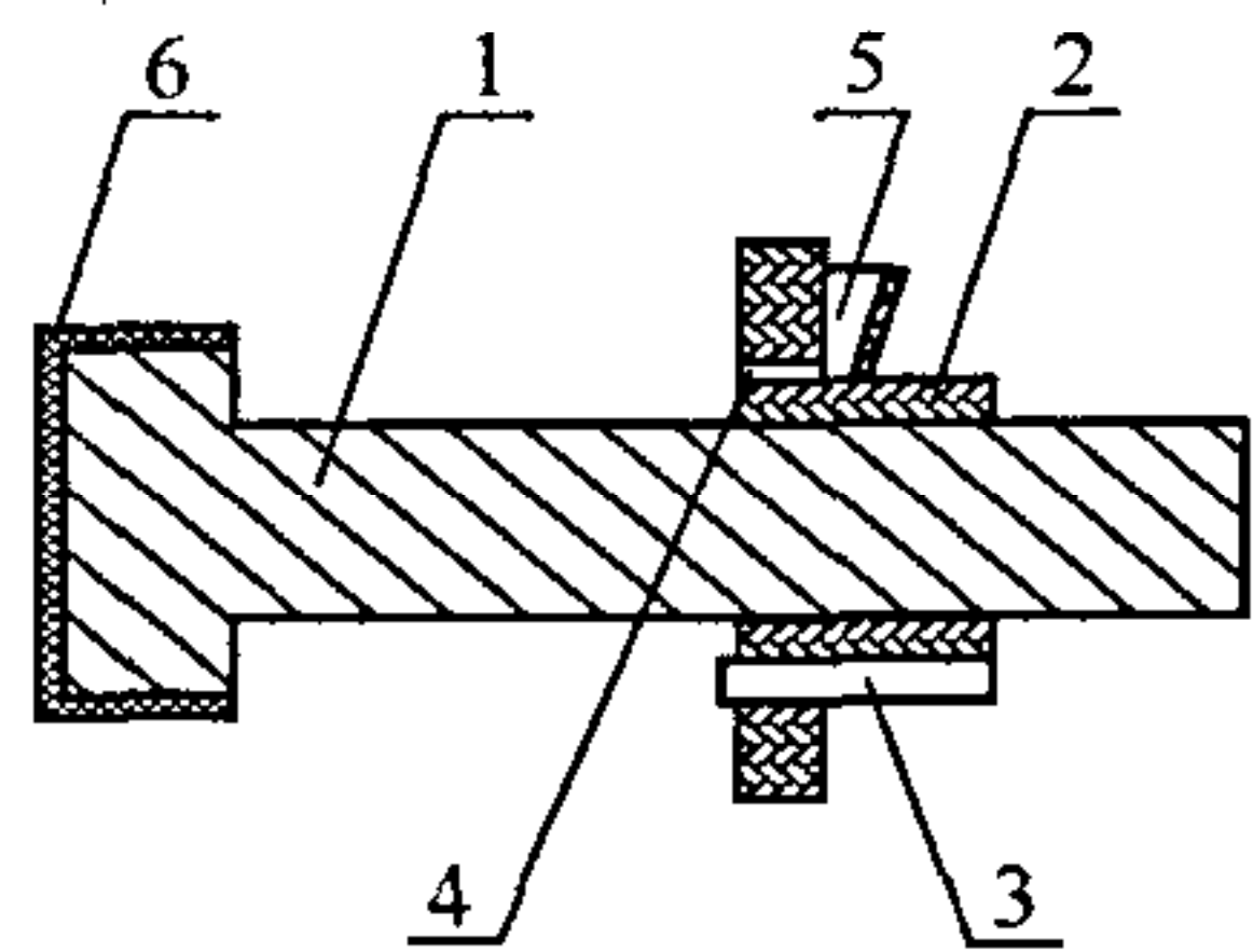
图 4.5.2 定位圆盘安装示意图
