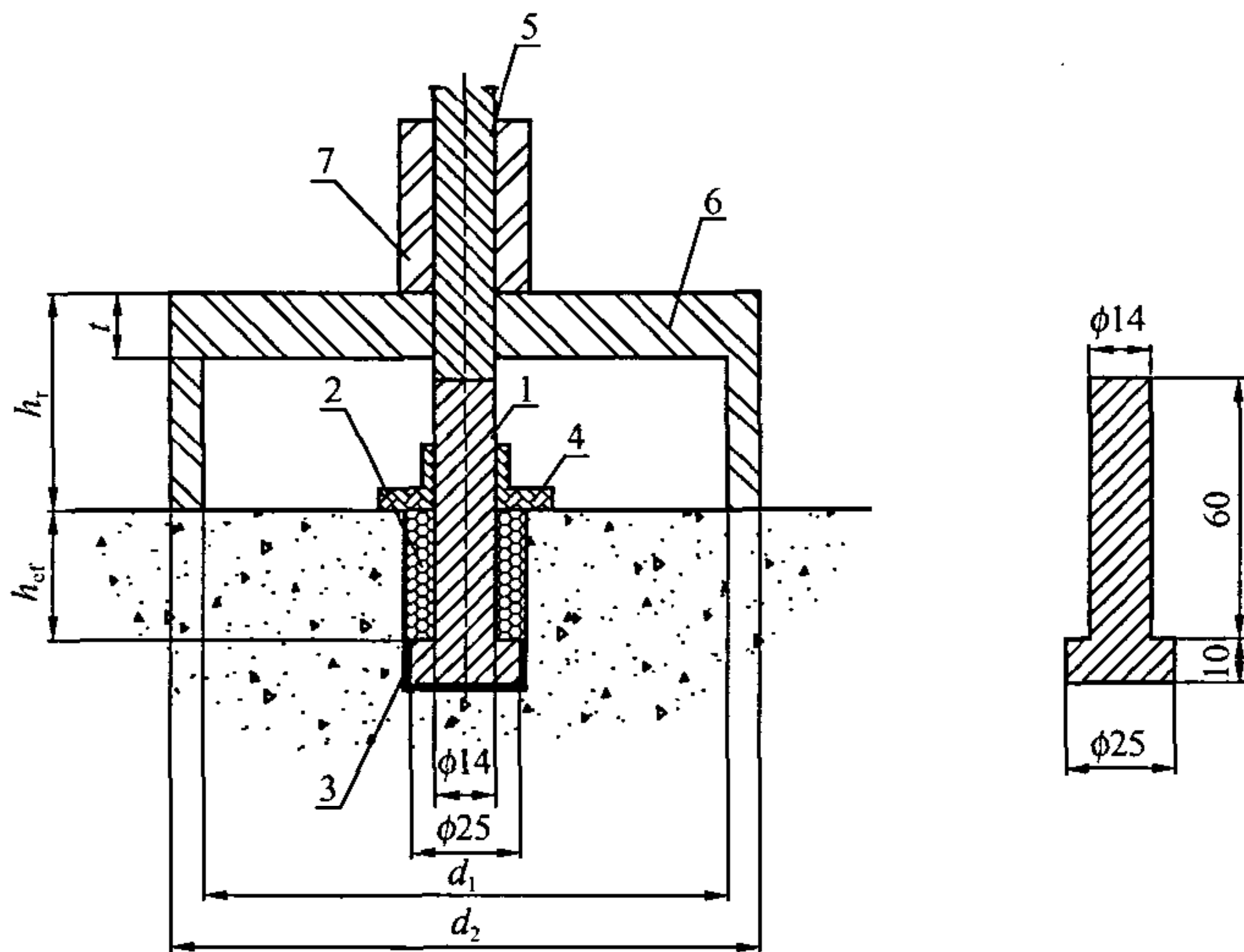
图 4.1.3 后锚固法试验装置示意图
