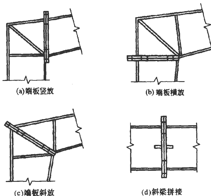
图 7.2.1 刚架斜梁的连接
