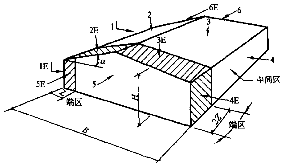
(a) 双坡刚架
