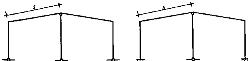
图 5.2.4 有摇摆柱的两跨刚架
