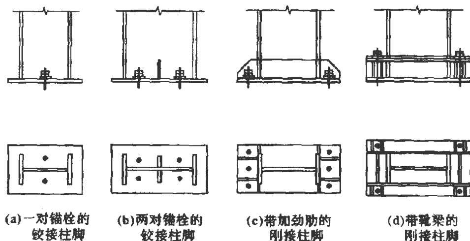
图 7.2.17 门式刚架轻型房屋钢结构的柱脚
