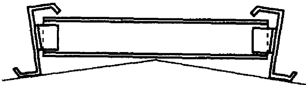
图 7.2.12 脊檩间的连系槽钢
