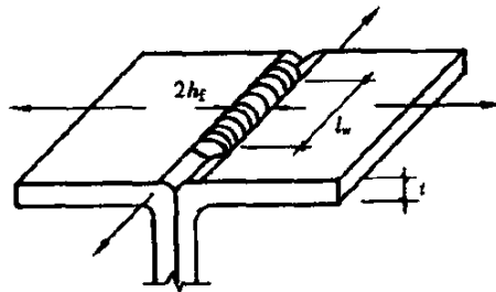
图 7.1.2-2 喇叭形焊缝
