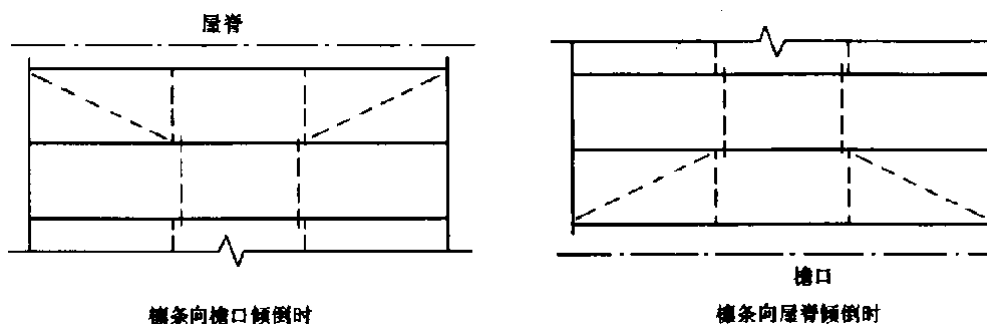
图 6.3.5 檩条间拉条的设置
