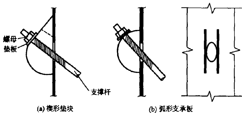
图 7.2.15 圆钢支撑的连接
