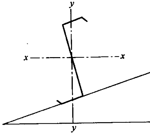
图 6.3.7 檩条的主轴
