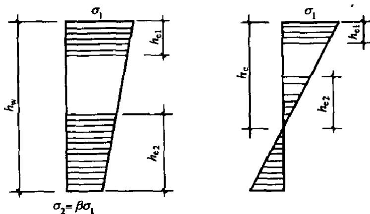
图 6.1.1 有效宽度的分布
