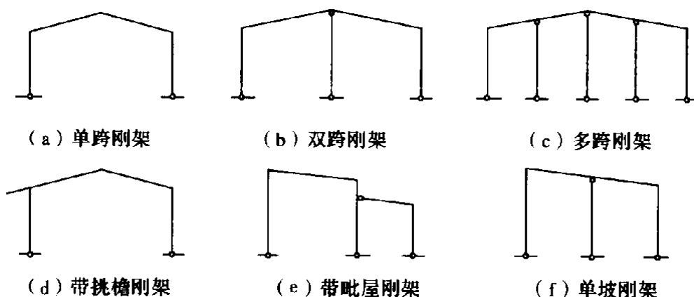
图 4.1.2 门式刚架形式示例
