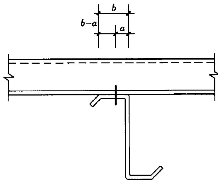
图 E. 0. 4 紧固件至转动中心的距离
