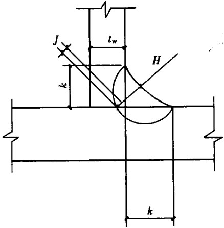
图 F.0.1 单面角焊缝
