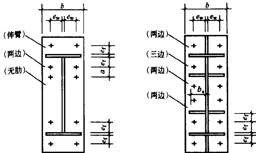
图 7.2.9 端板的支承条件
