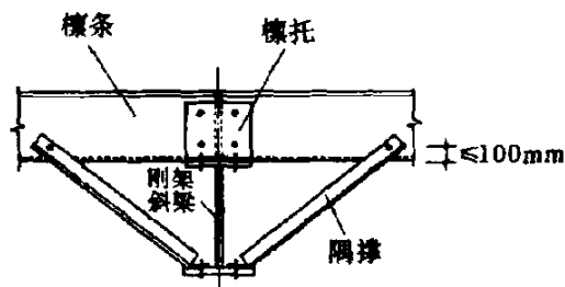
图 7.2.14 隅撑的连接
