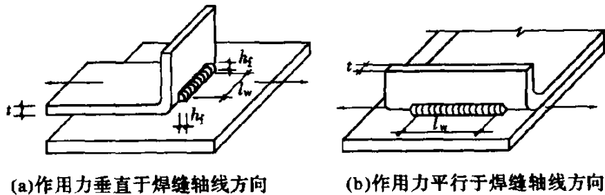
图 7.1.2-1 单边喇叭形焊缝
