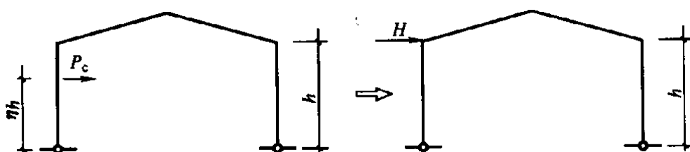
图 5.2.3-2 刚架在吊车水平荷载作用下柱顶的等效水平力
