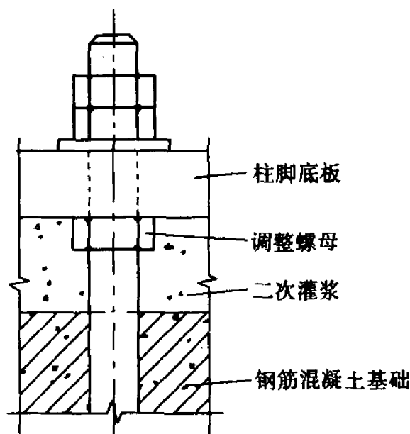
图 8.2.5 柱脚的安装
