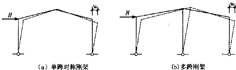
图 6.1.3-2 一阶分析时的柱顶侧移
