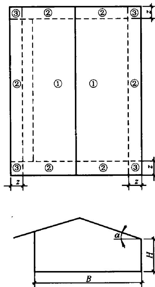
图 A.0.2-3 挑檐的风荷载体型系数分区
