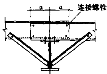
图 7.2.13 斜卷边檩条的搭接
