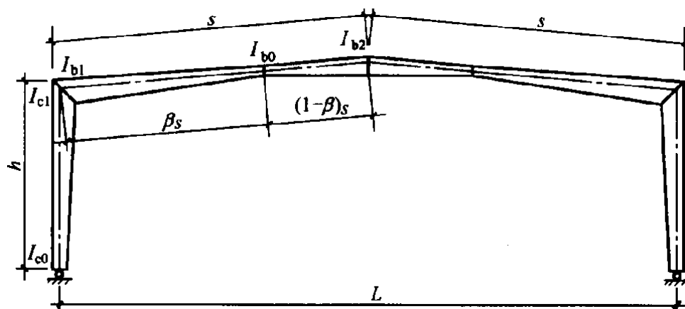
图 5.2.1 变截面刚架的几何尺寸
