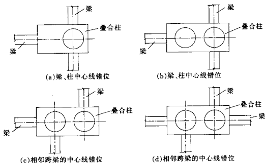
图 8.2.2 中心线错位情况下梁柱连接方式
