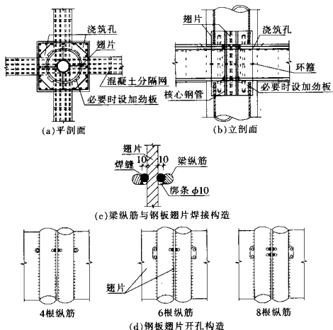
图 8.2.5 钢板翅片转换型连接节点构造
