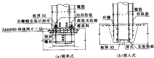
图 8.4.1 叠合柱的柱脚构造
