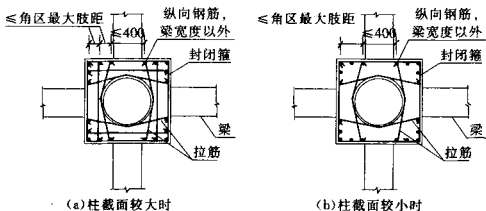
图 6.2.18 钢管混凝土叠合柱的配箍方式
