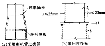
图 8.1.3 不等直径钢管接长的构造
