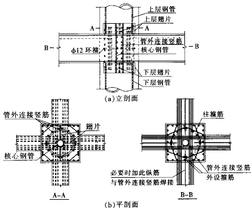
图 8.2.6 钢管钢筋转换型连接节点构造
