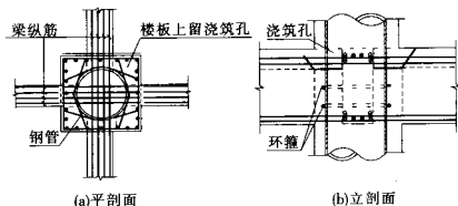
图 8.2.4 钢管贯通型连接节点构造
