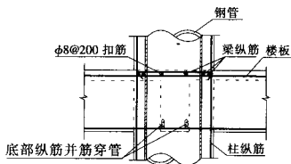
图 8.2.3 梁纵筋布置方式
