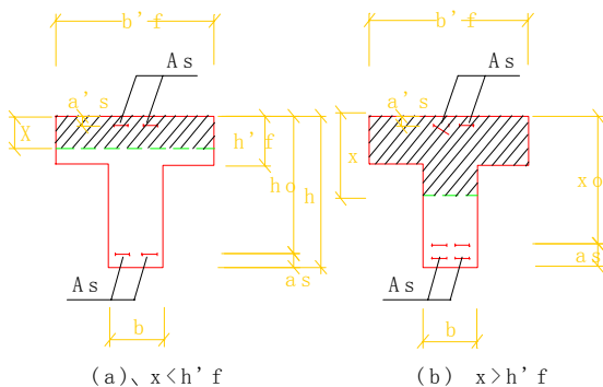
图4.0.2 T形截面受弯构件受压区高度位置
