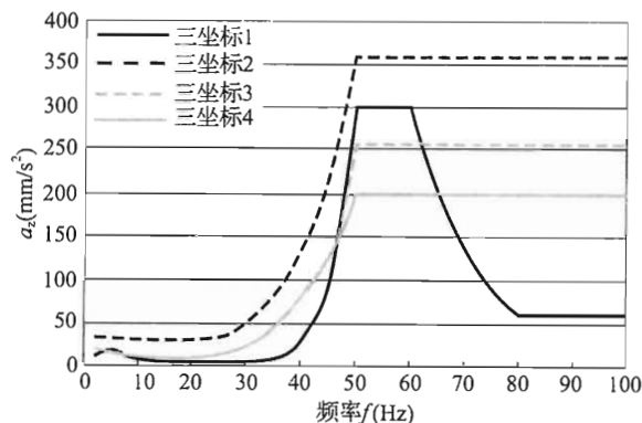
图 2 三坐标测量机的容许振动值
