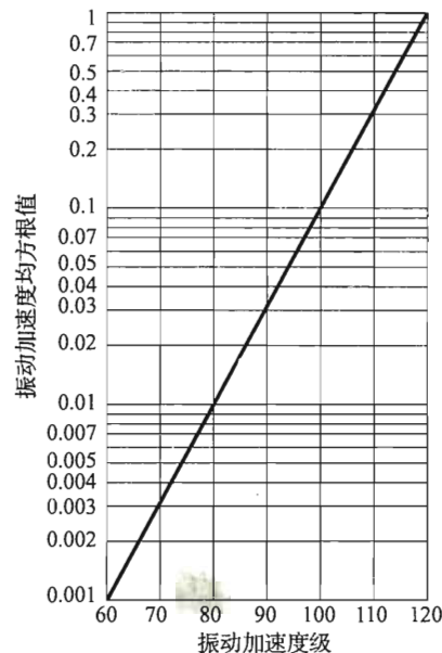
图 5 振动加速度级和振动加速度均方根值之间的关系
