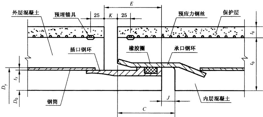
b) PCCPSE 管子接头图
