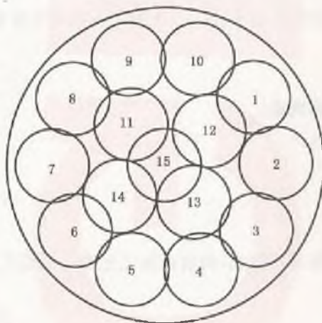
图 1 第一层捣压位置示意图
