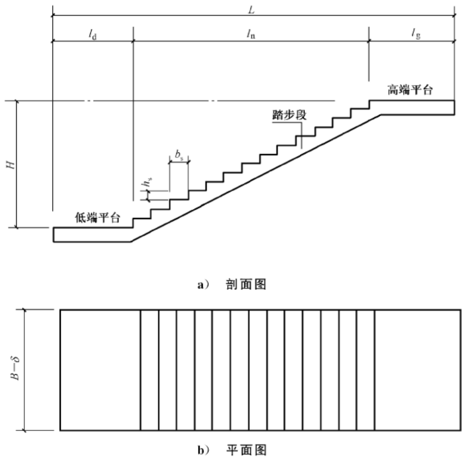
图 1 预制楼梯示意图
