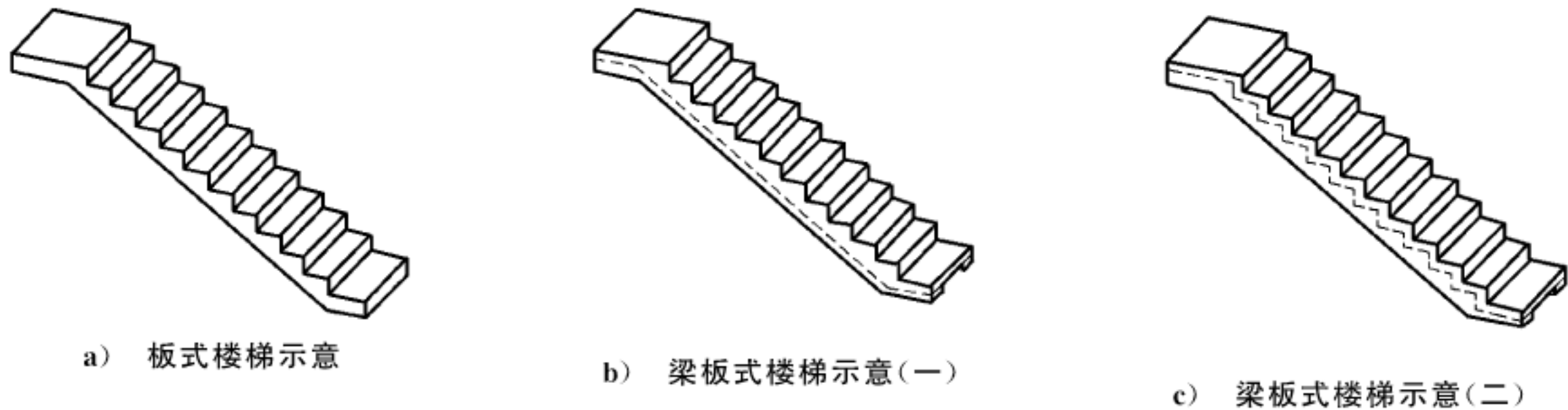
图 1 预制楼梯示意图
