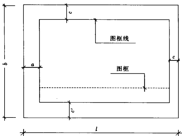
图 2.12.2 规格幅面图纸的尺寸示意
