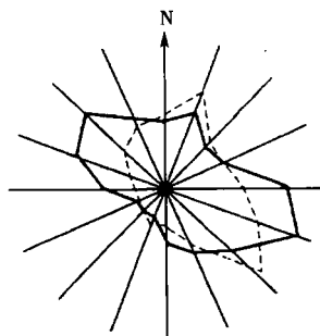
图 2.4.6 结合风象玫瑰图标绘的指北针
