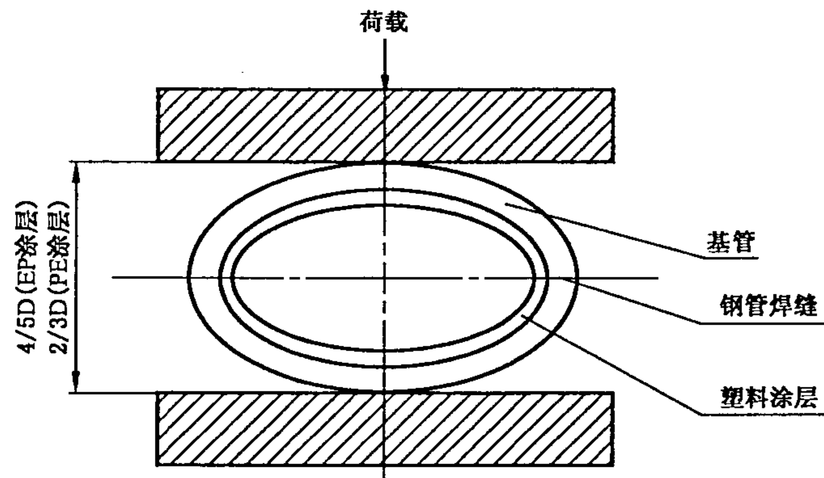
图 5 压扁试验
