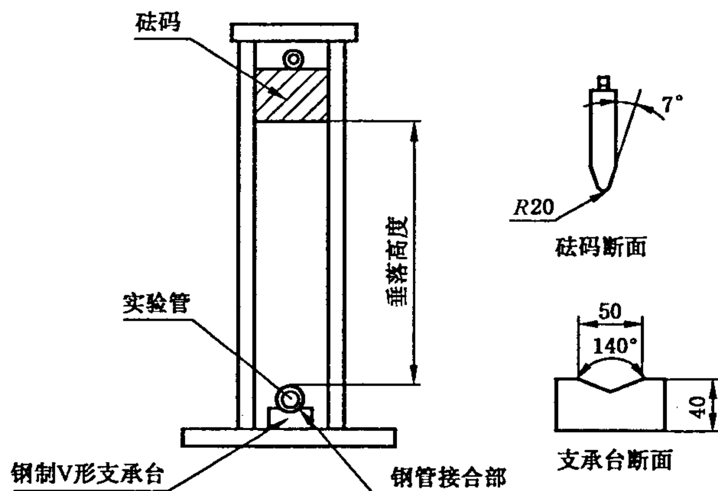
图 6 冲击试验
