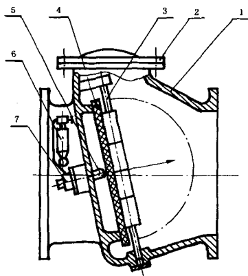
1—阀体;2—阀盖;3—阀轴;4—阀瓣(双); 5—活塞(双);6—节流阀;7—缓闭装置
