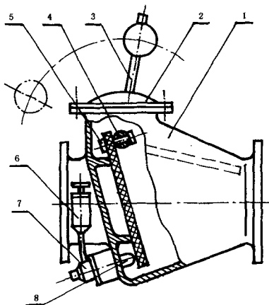
1—阀体;2—阀盖;3—重锤;4—阀轴;5—阀瓣; 6—节流阀;7—缓闭装置;8—活塞
