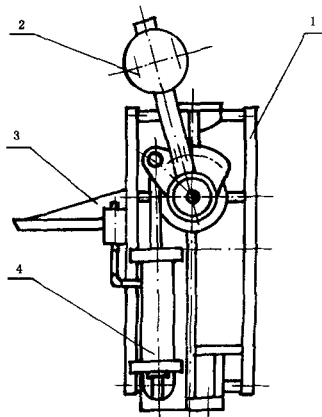
1—阀体;2—重锤;3—瓣板;4—缓闭装置
