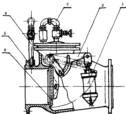
1—缓闭装置;2—扇形臂和连杆;3—阀后补气装置; 4—阀前补气装置;5—阀体;6—阀瓣
