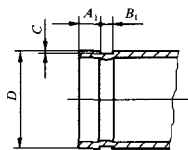
图 14 钢管滚槽结构图
