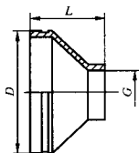
图 12 异径管(螺纹式)结构图
