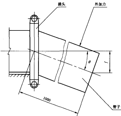
图 18 转角检查装置原理图
