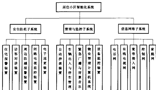
图2 居住小区智能化系统功能框图
