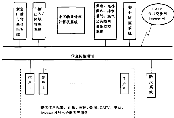
图 1 居住小区智能化系统总体框图
