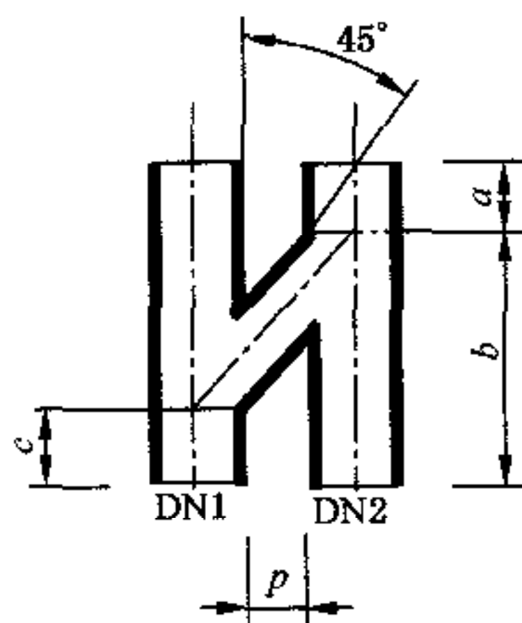
图 19 H 管
