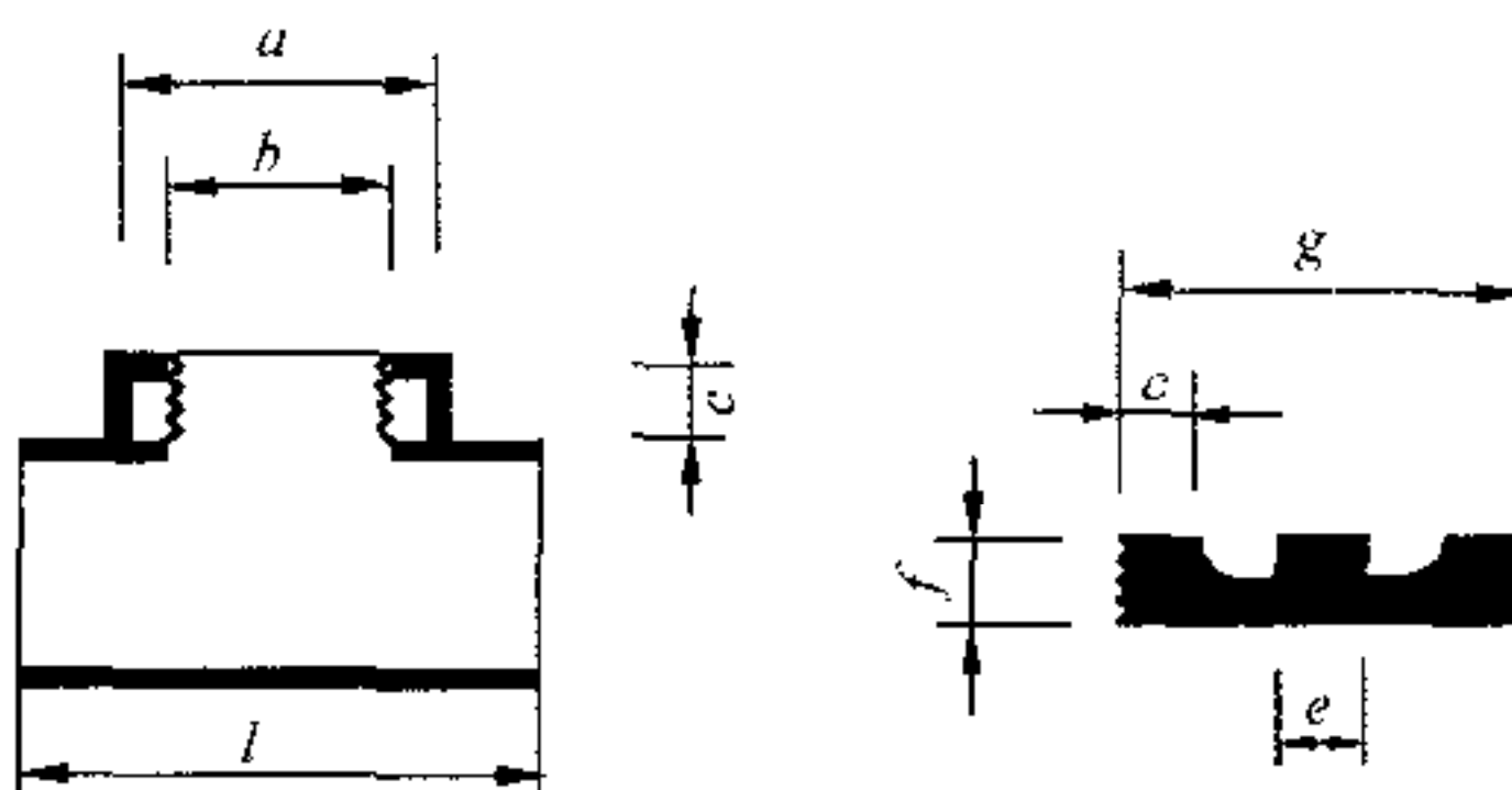
图 25 横式清扫口
