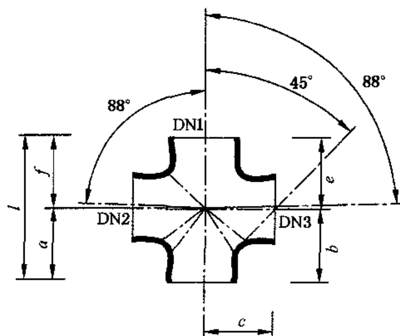
图 14 88°四通
