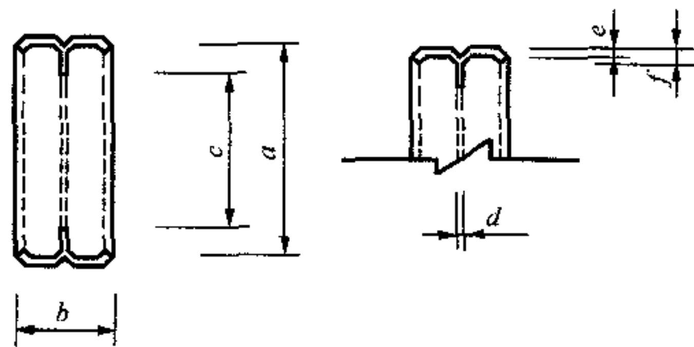
图 33 拉锁型橡胶密封圈 表 33 拉锁型橡胶密封圈规格尺寸
