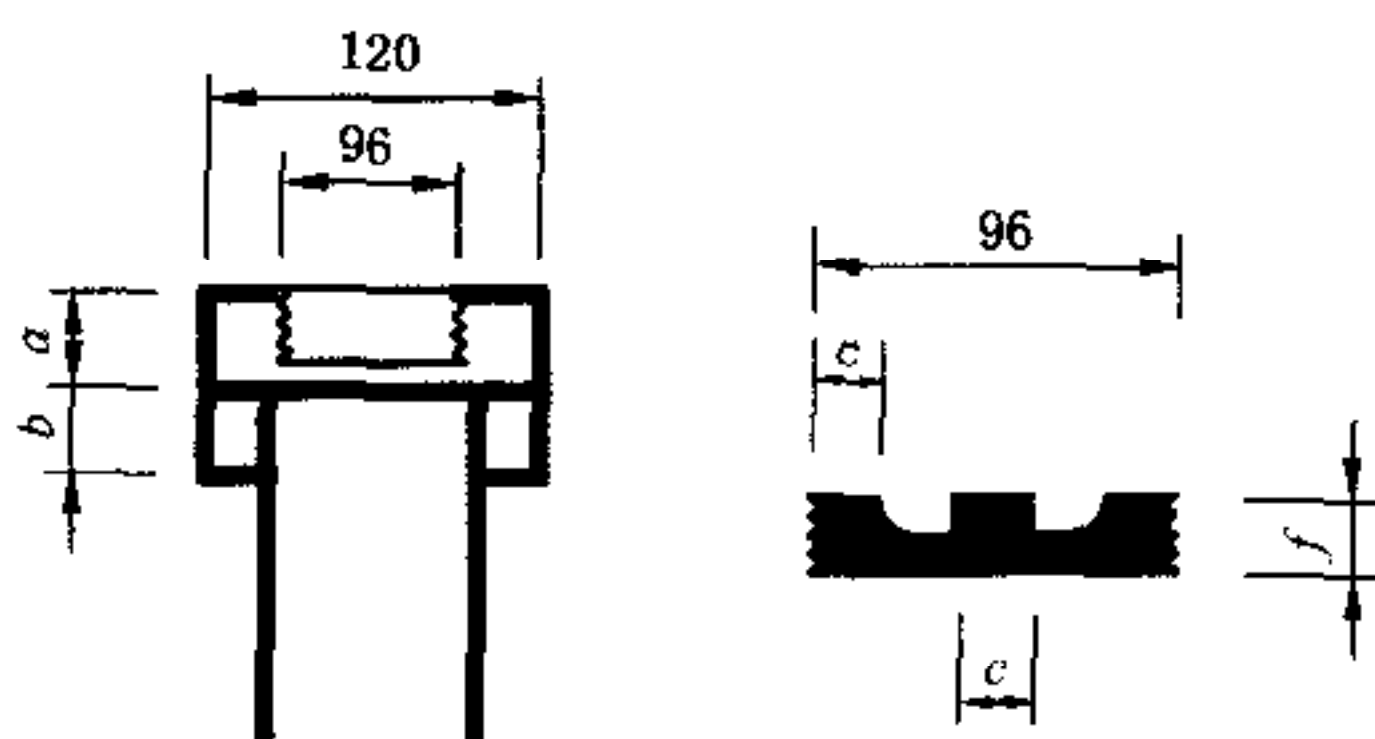
图 24 直式清扫口
