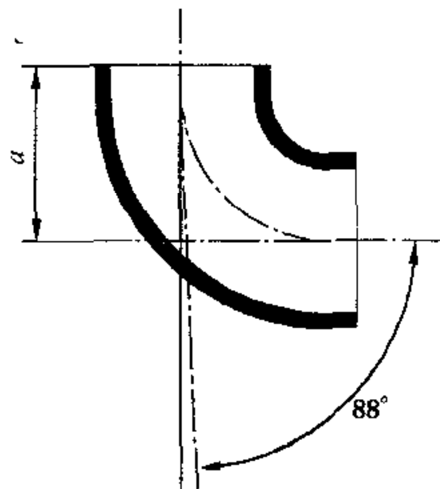
图 4 88°弯头
