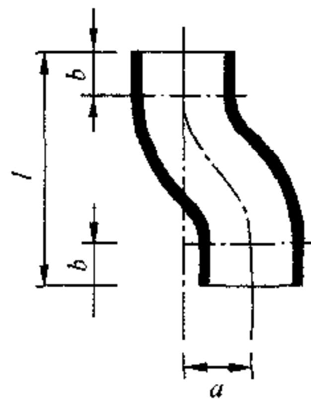
图 5 乙字弯头
