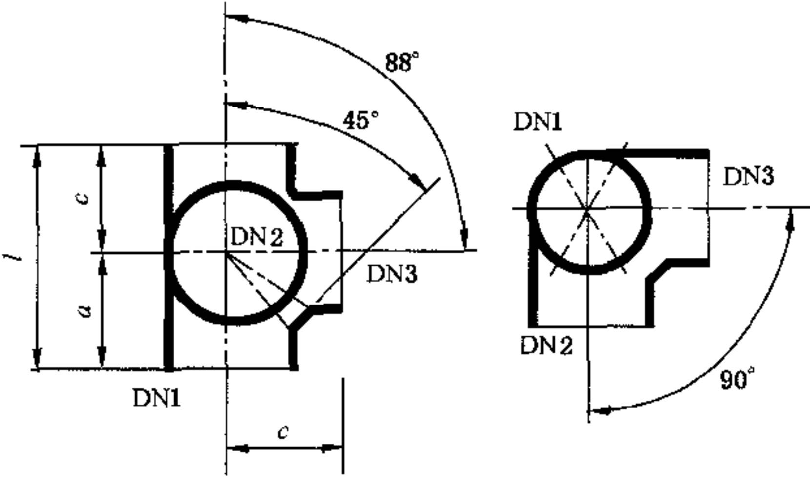
图 13 88°直角四通
