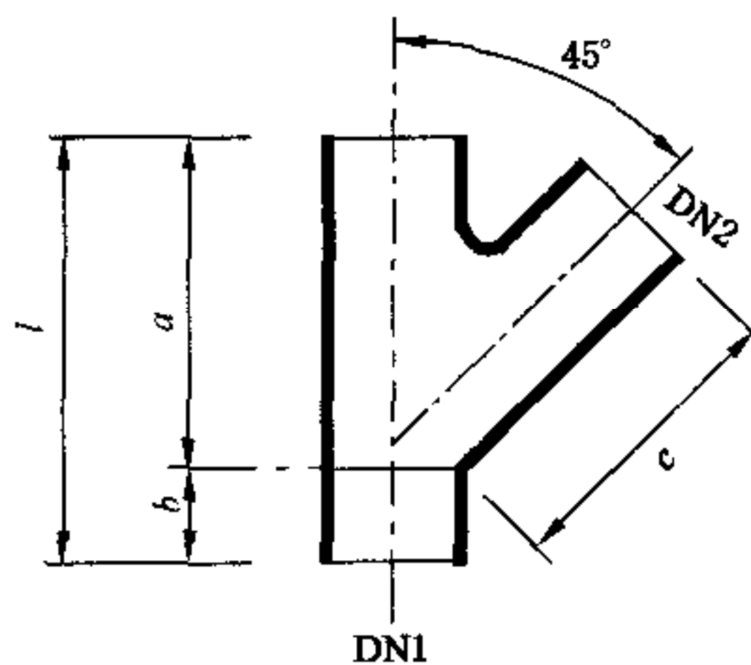
图 10 45°三通
