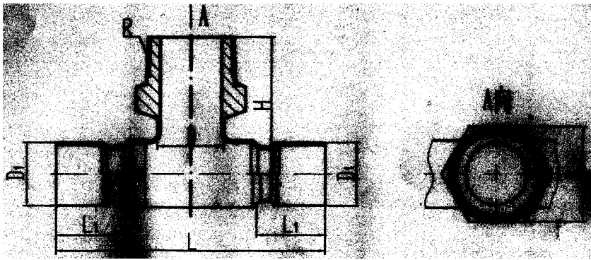
图A.9 外螺纹转换三通
