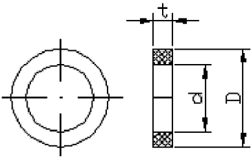
图B.3 螺母移动转换接头用密封圈 表B.3 螺母移动转换接头用密封圈尺寸 mm
