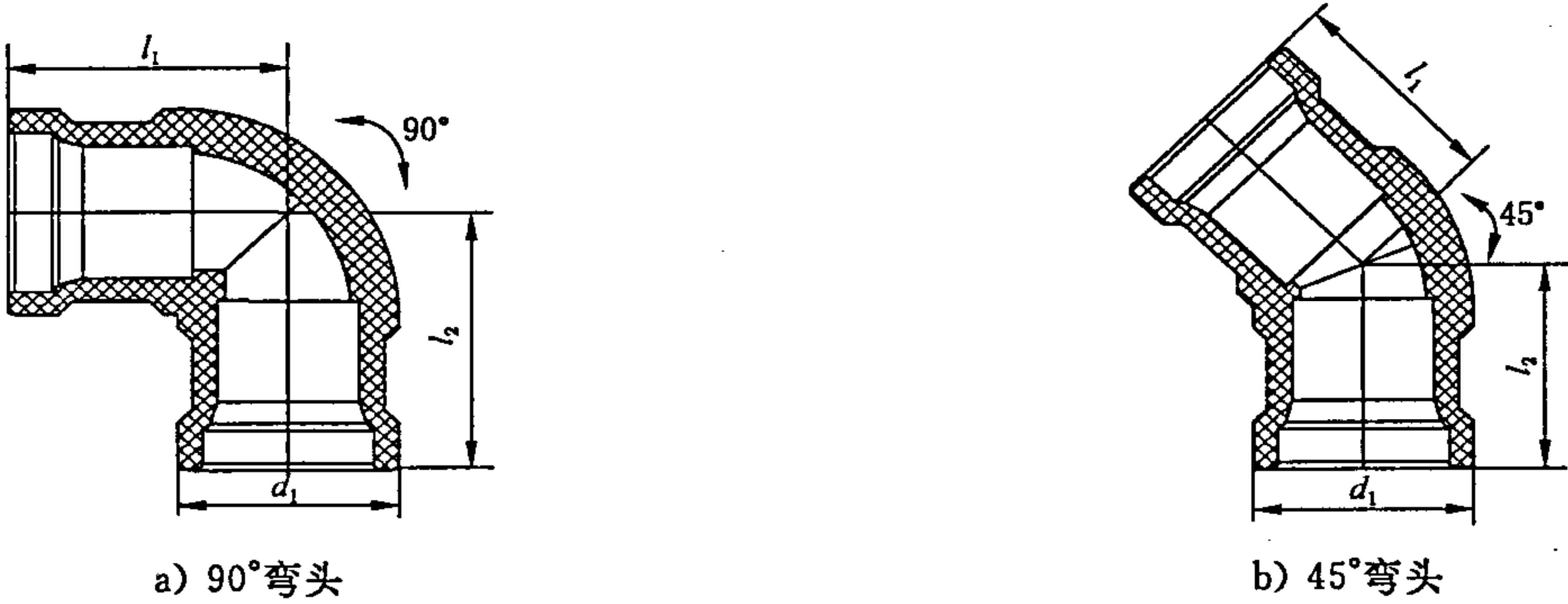
图 A.3 弯头 表 A.3 弯头尺寸
