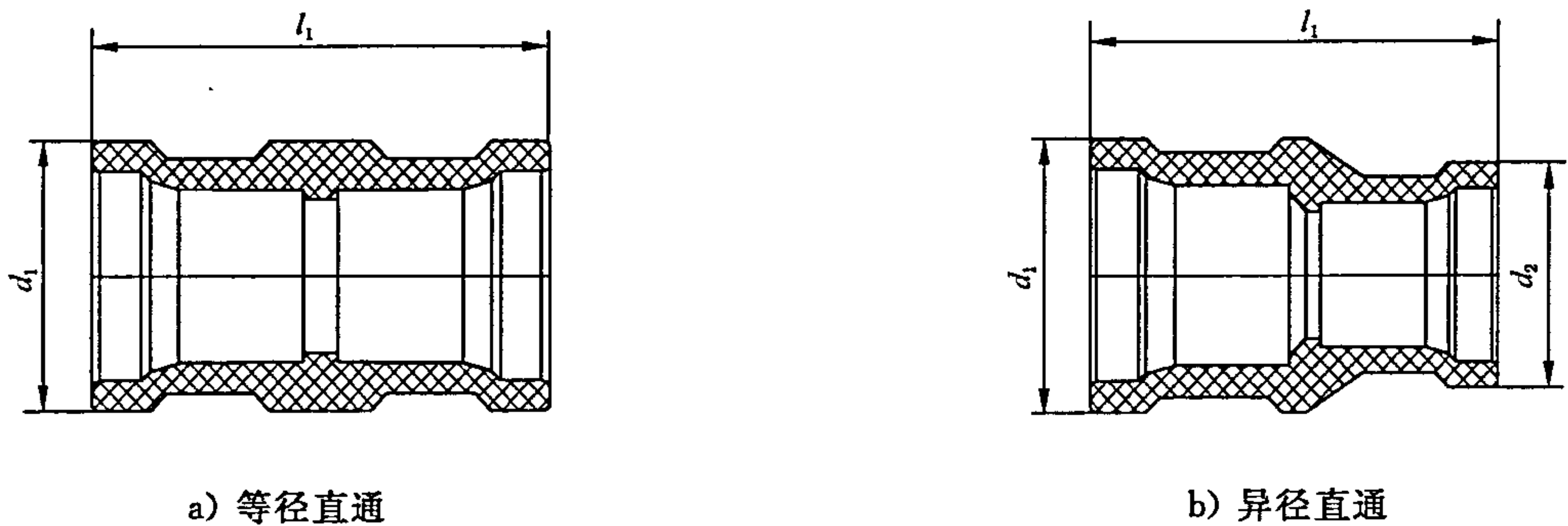
图 A.1 直通 表 A.1 直通尺寸 单位为毫米
