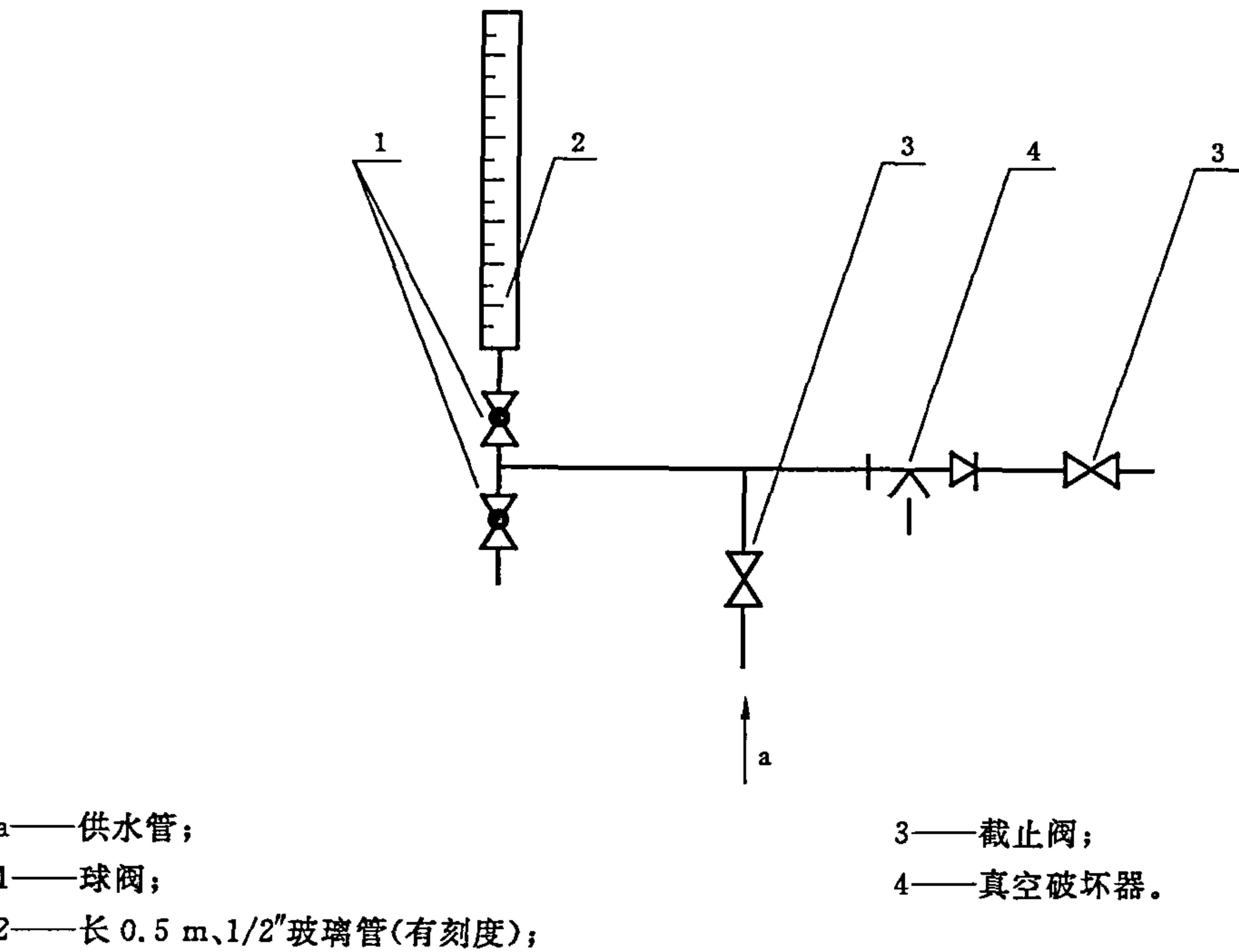
图 3 止回阀关闭压力性能试验装置
