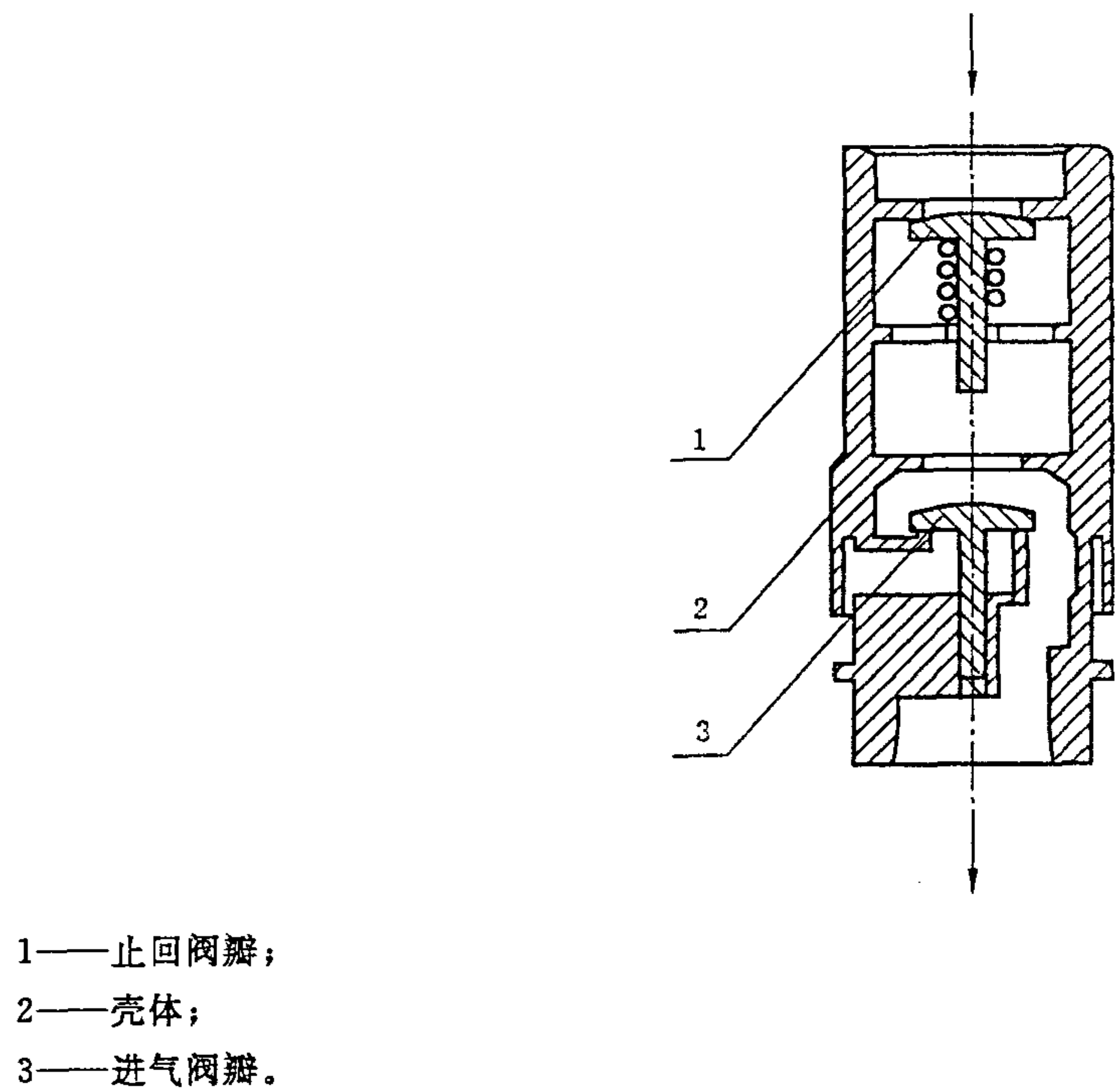
图 B.4 软管型
