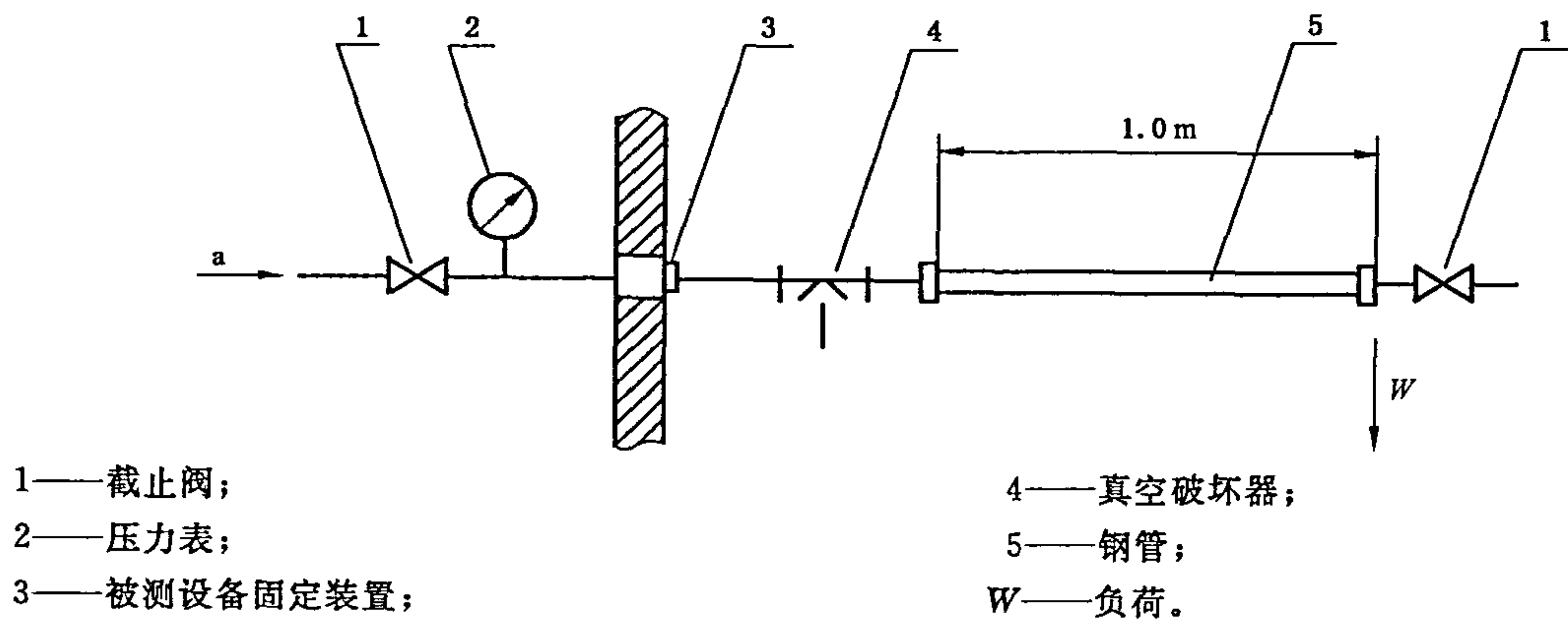
图 1 弯曲强度试验装置
