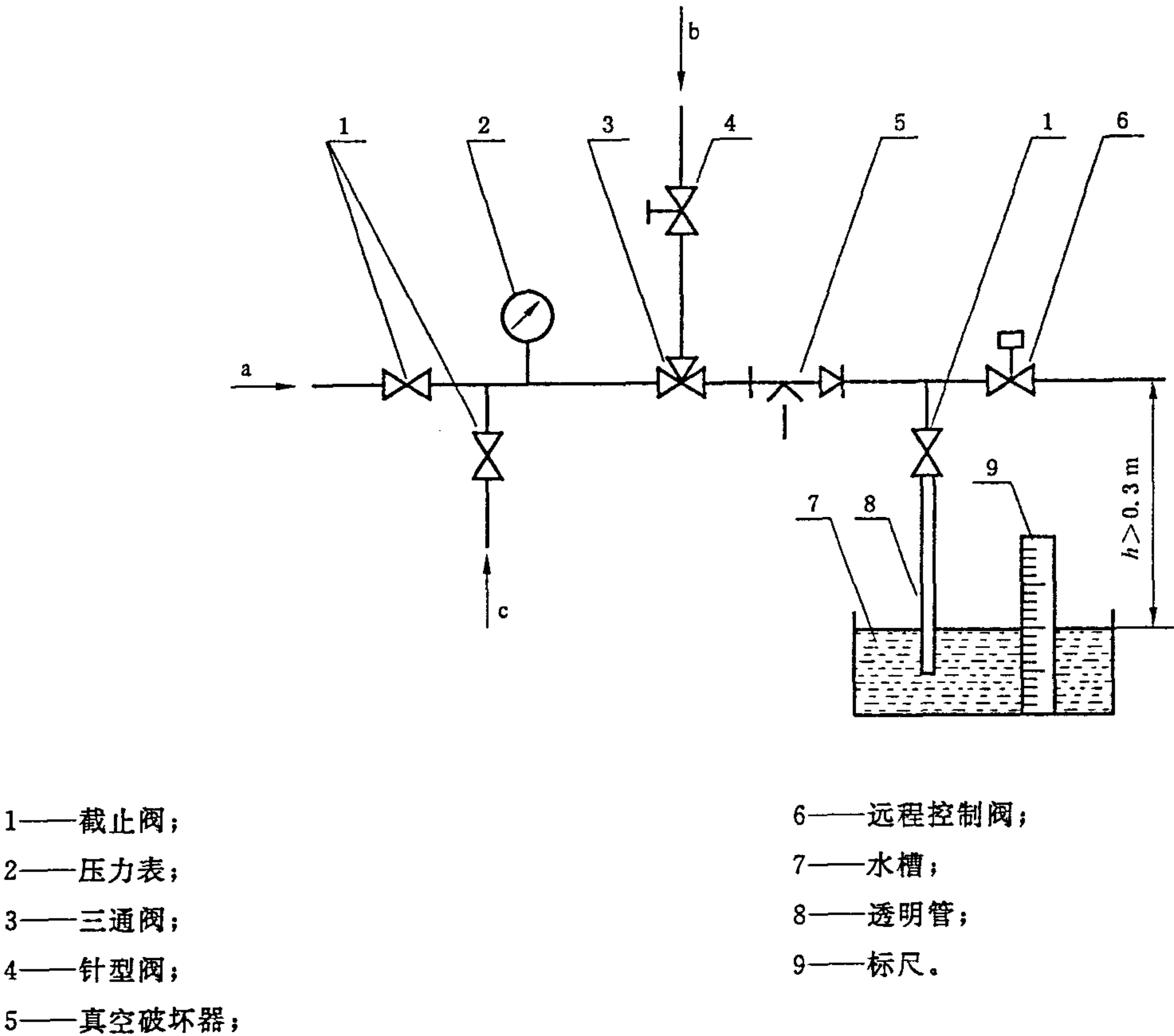
图 4 进气阀开启性能/耐久性能试验装置
