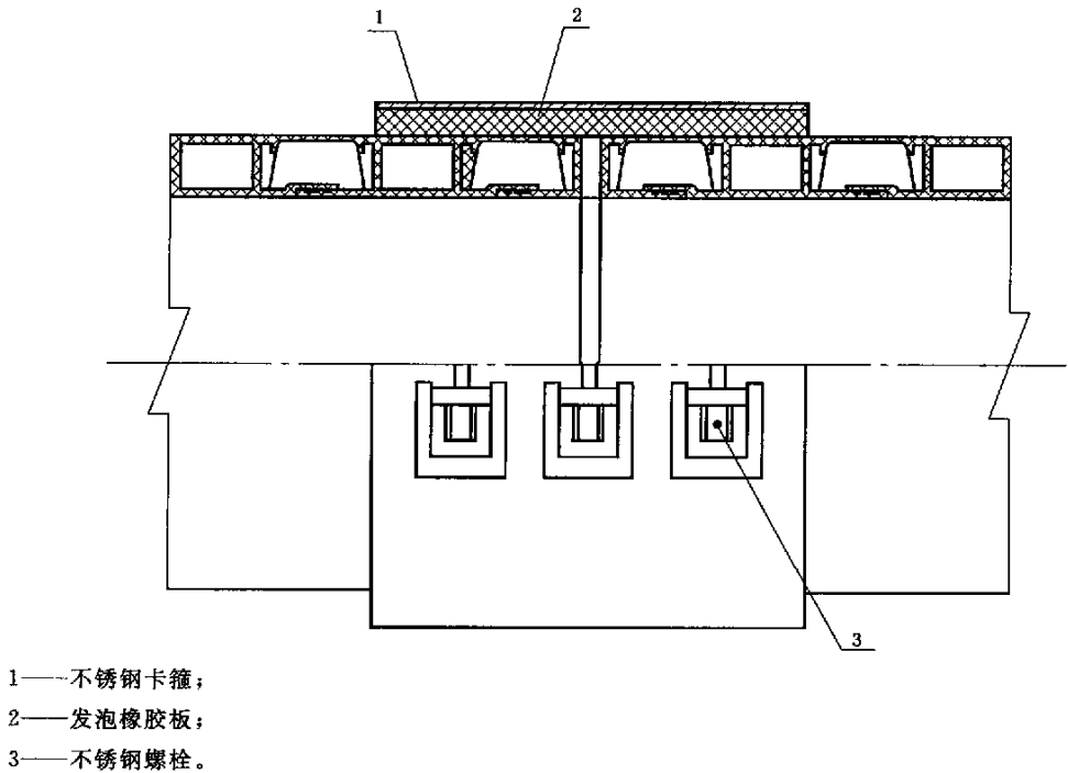
图 A.1 卡箍式弹性连接方式示意图
