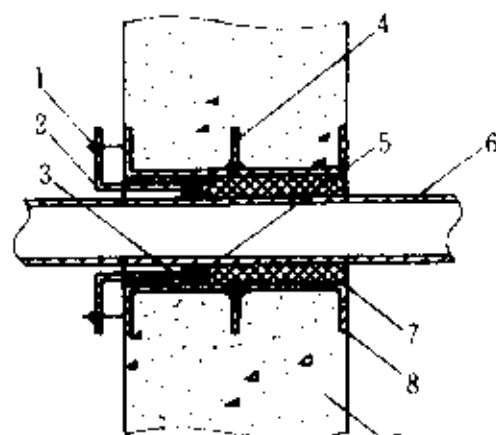
图 9.5.2-2 套管式穿墙管构造图
