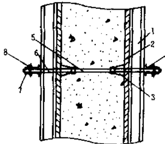
图 5.6.3 模板拉杆螺栓连接图
