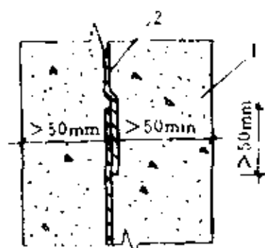
图 9.2.10-2 遇水膨胀胶条 搭接平面图
