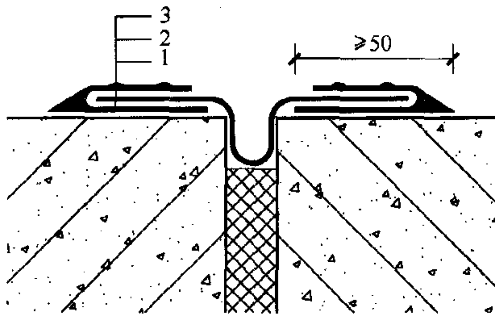
图 4.2.5-1 粘贴内置式密封止水带
