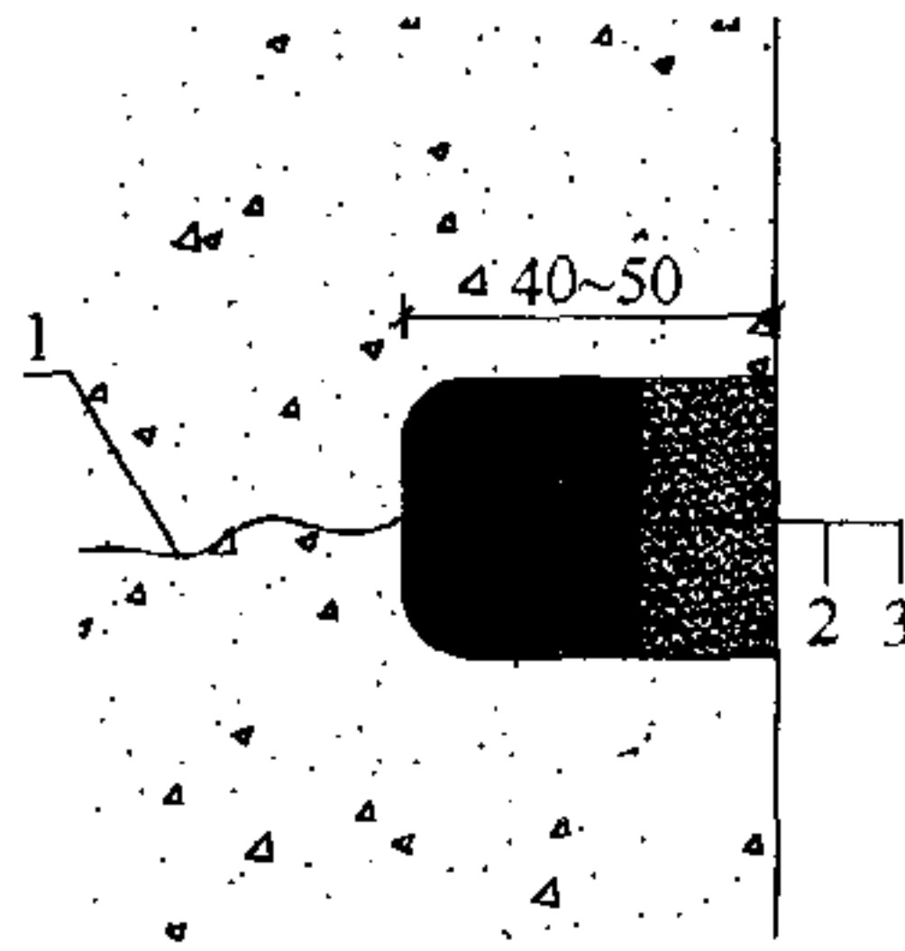
图 4.2.1-3 裂缝快速封堵止水
