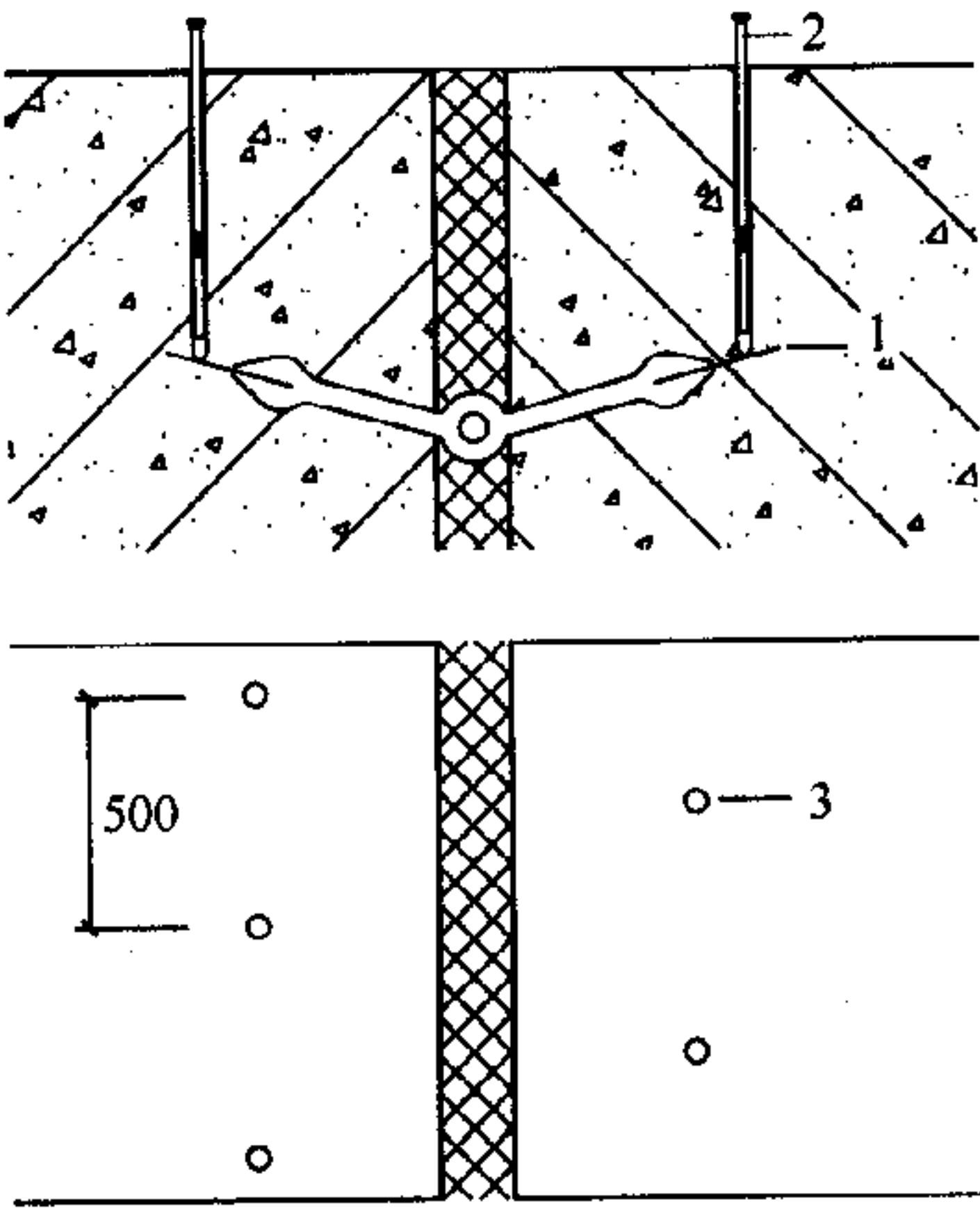
图 4.2.4-2 钻孔至止水带两翼 钢边并注浆止水
