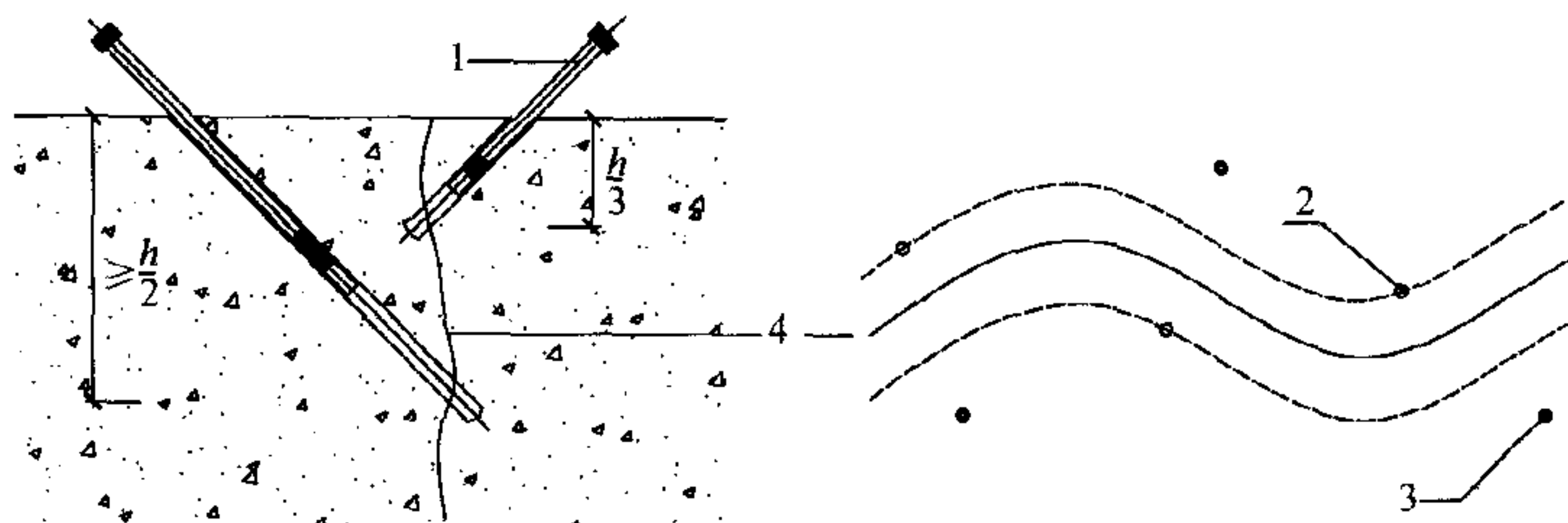
图 4.2.1-2 钻孔注浆止水及补强的布孔
