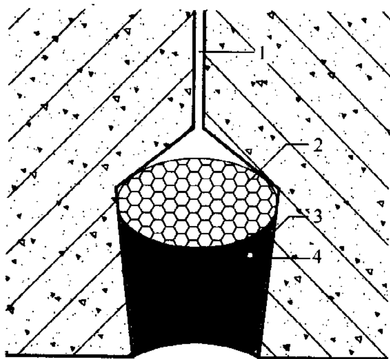
图 5.2.2 拱顶管片环(纵)缝嵌缝
