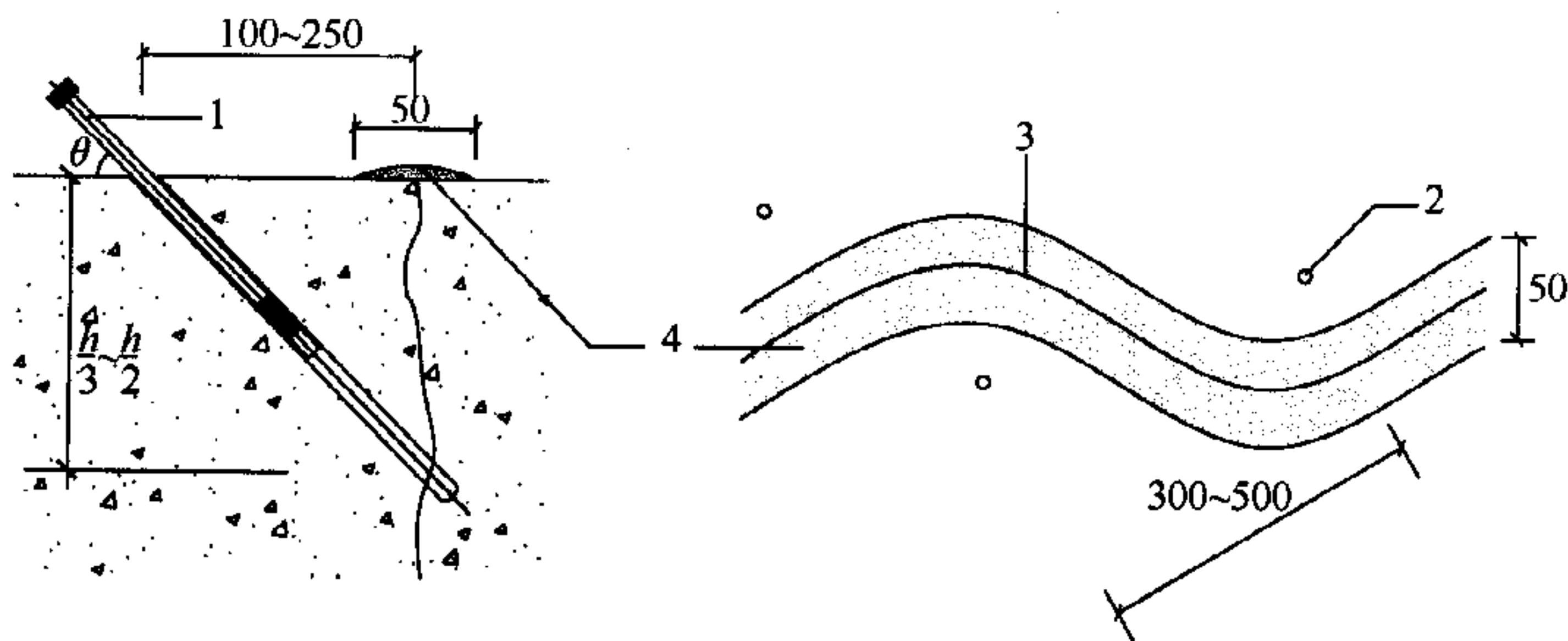
图 4.2.1-1 钻孔注浆布孔
