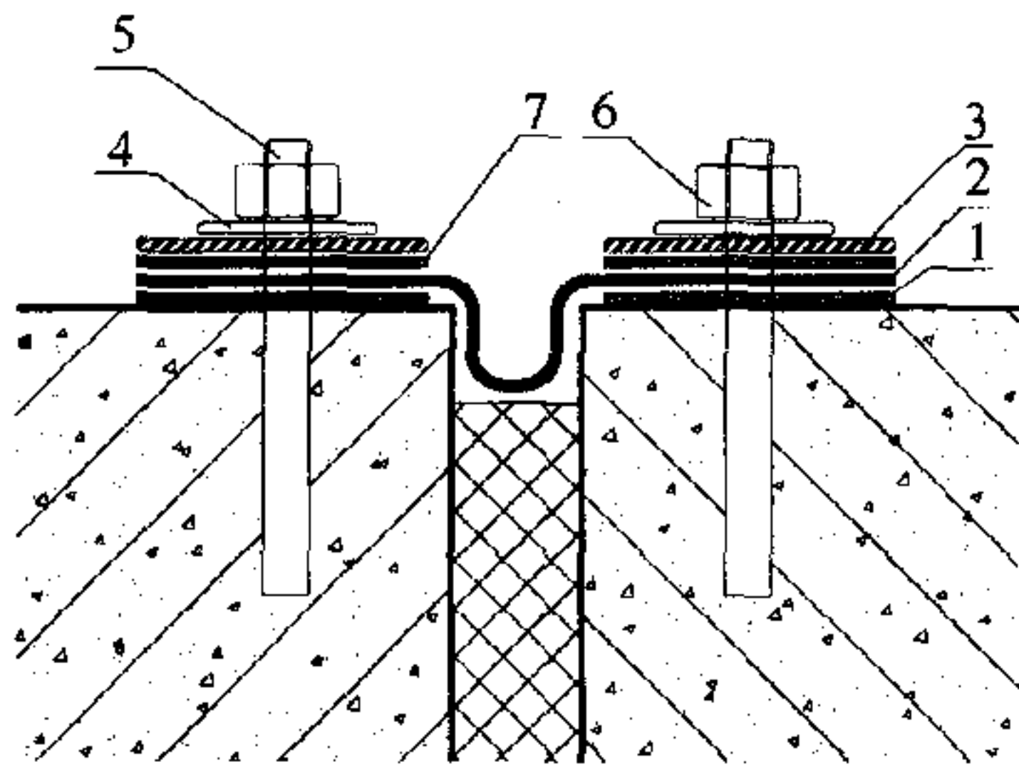
图 4.2.5-2 螺栓固定内置式密封止水带
