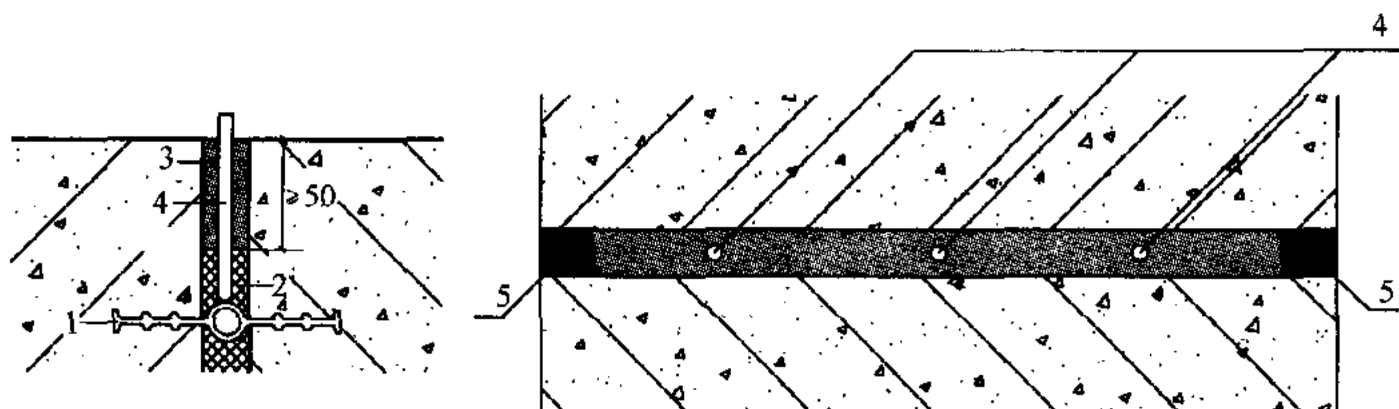
图 4.2.4-3 变形缝埋管（嘴）注浆止水
