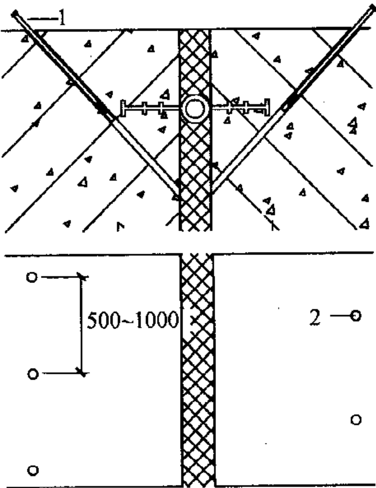
图 4.2.4-1 钻孔至止水带迎水面 注浆止水
