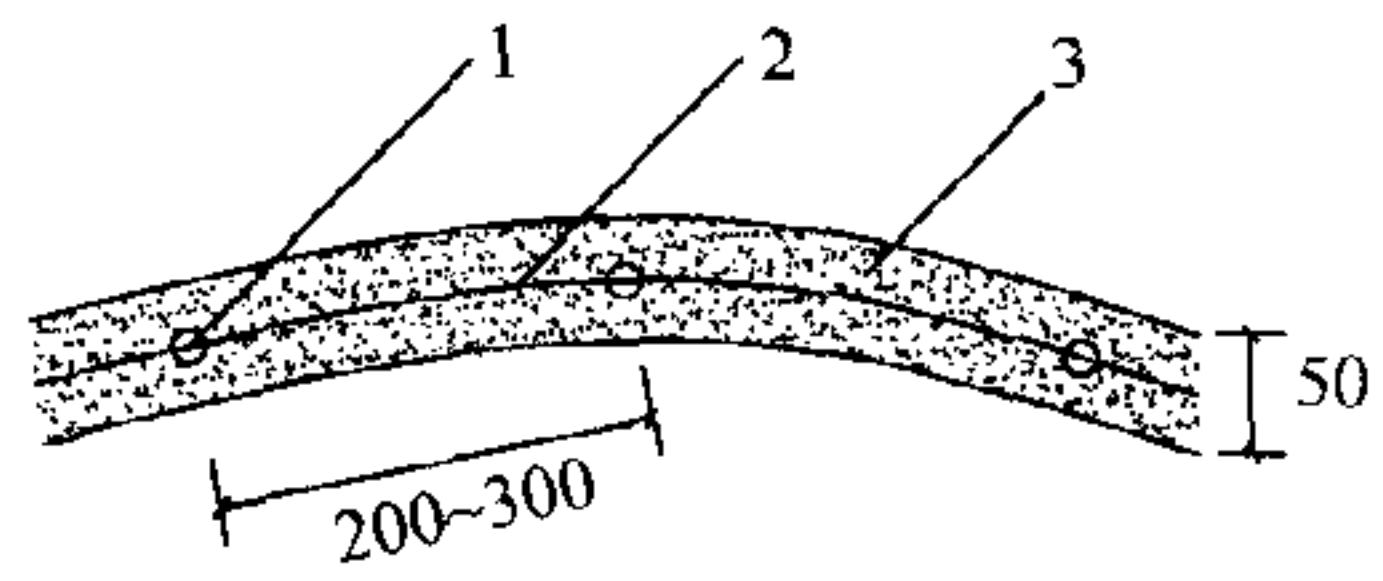
图 4.2.1-4 贴嘴注浆布孔
