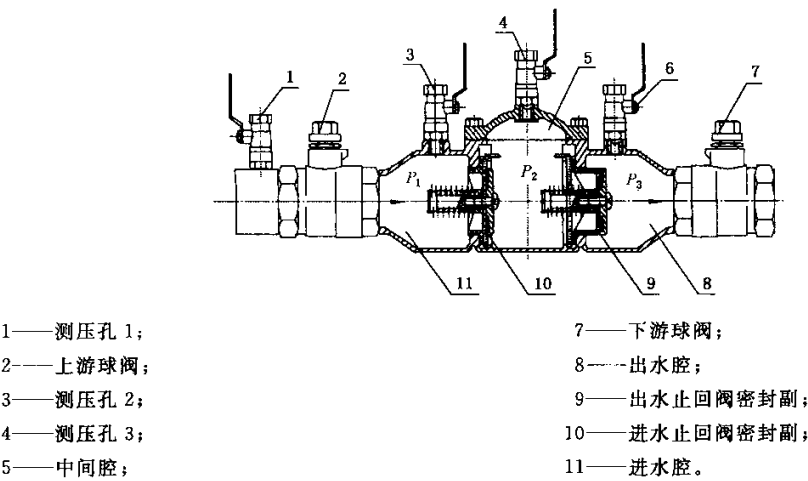
图 A.2 螺纹连接升降式双止回阀倒流防止器结构示意图
