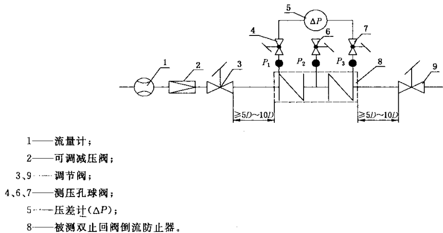
图 2 压力损失试验装置示意图
