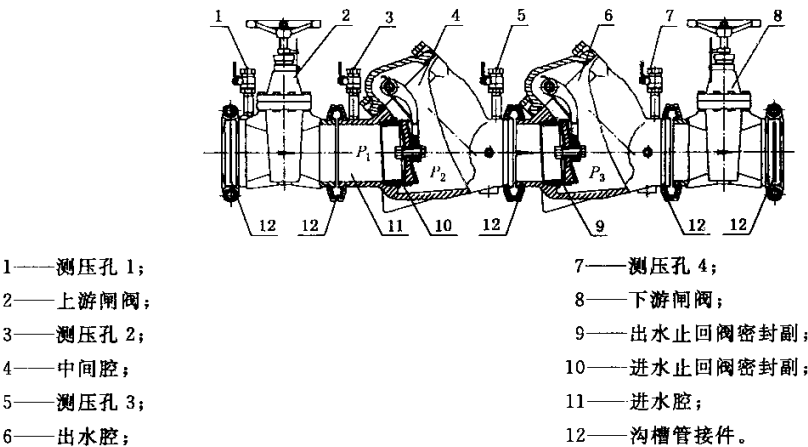
图 A.3 沟槽连接旋启式双止回阀倒流防止器结构示意图
