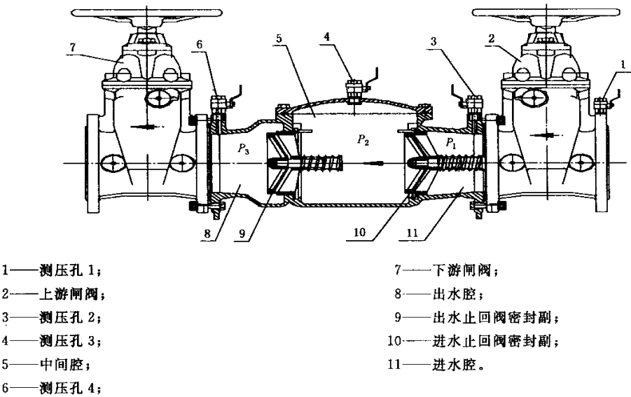
图 A.1 法兰连接升降式双止回阀倒流防止器结构示意图
