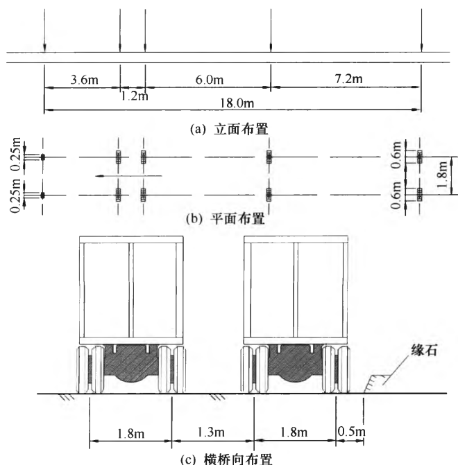
图 10.0.2-2 城—A 级车辆荷载立面、平面、横桥向布置
