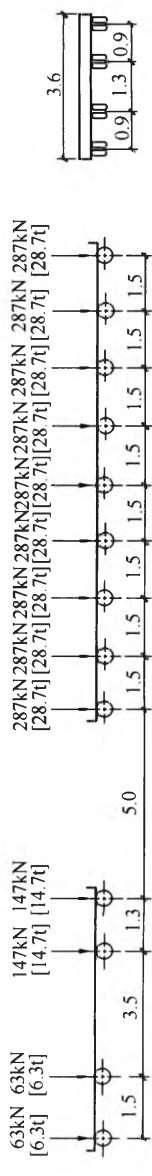
挂车纵向排列
