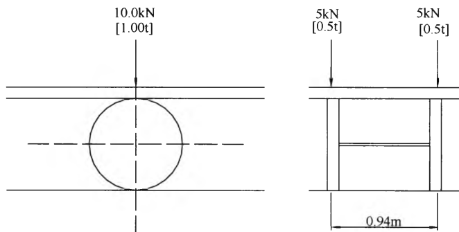
图 10.0.6 一辆人力劳动车荷载图
