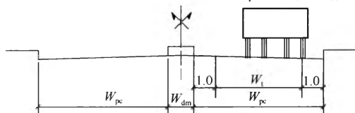
图 A.0.2-3 ( W_{pc} = 2 车道路面宽)
