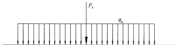
图 10.0.2-1 车道荷载
