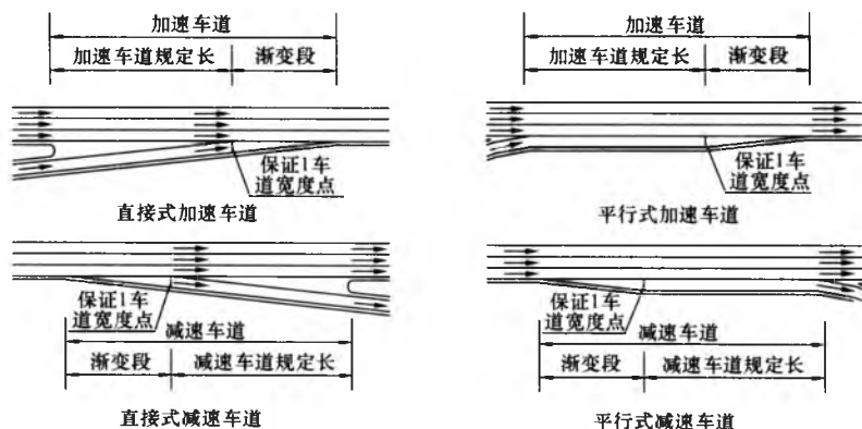
图 7.3.1-1 变速车道
