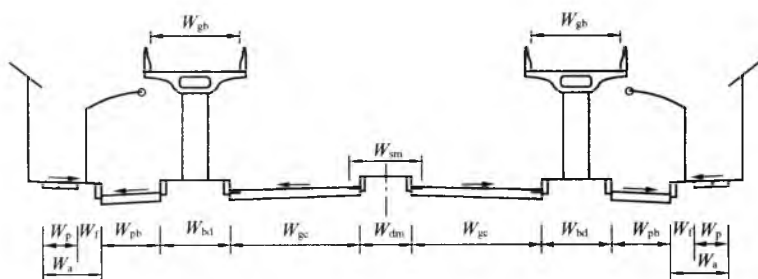
图 5.2.3-5 分离式高架道路横断面
