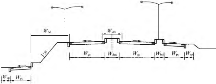
图 5.2.2 地面整体式横断面（郊区型）
