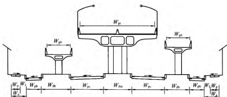
图 5.2.3-2 整体式高架道路有匝道路段横断面
