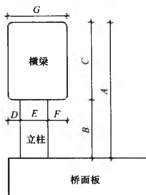
图 6 钢筋混凝土梁柱式护栏（单位：cm）
