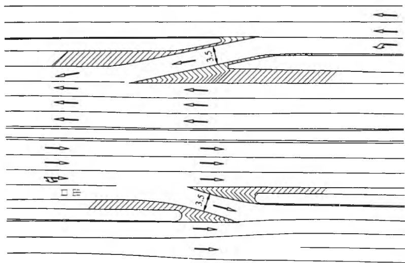
图 7.1.3 主辅路出入口设置图
