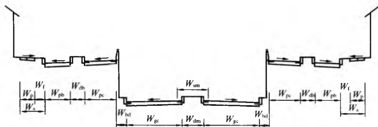
图 5.2.4 路堑式横断面
