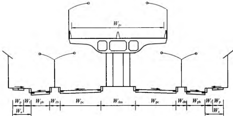
图 5.2.3-1 整体式高架道路无匝道路段横断面
