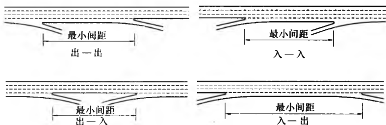
图 1 出入口类型
