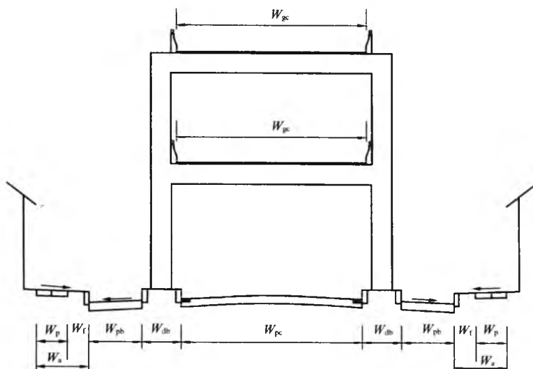
图 5.2.3-3 分离式高架道路无匝道路段横断面
