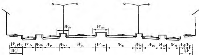
图 5.2.1 地面整体式横断面（城区型）
