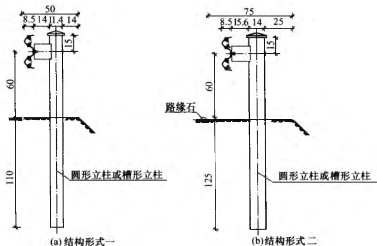
图 2 路侧波形梁护栏（单位：cm）
