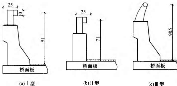
图 8 组合式桥梁护栏 (单位: cm)
