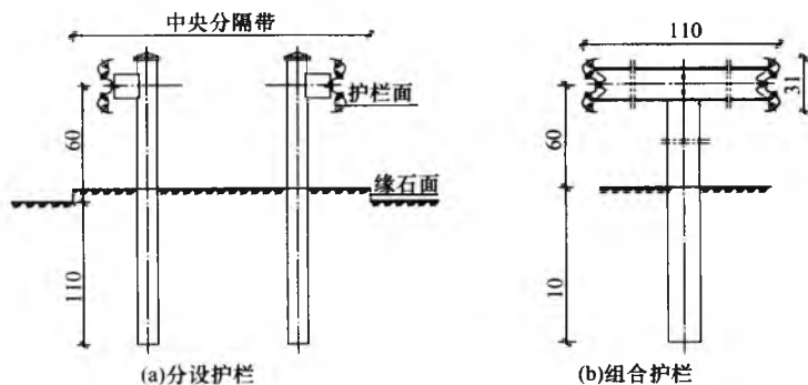
图3 路中波形梁护栏 (单位: cm)
