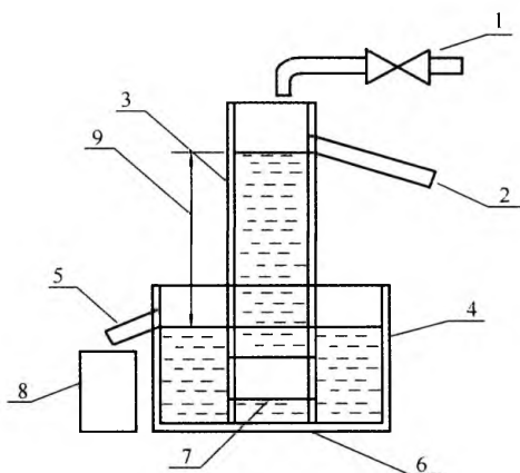
图 A.0.1 透水系数试验装置示意图
