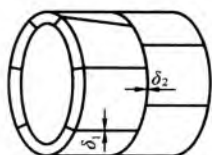
图 4 管片拼装缝隙位置示意
