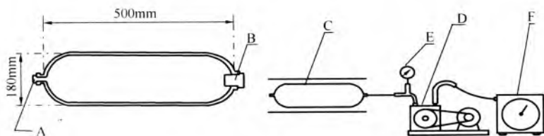
图 4.5.4-2 采样瓶（左）与真空处理装置（右）
