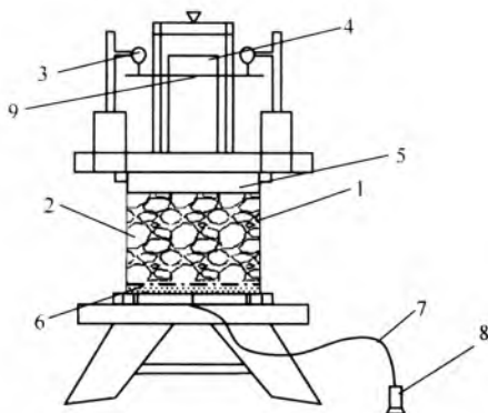
图 6.4.2 蠕变仪
