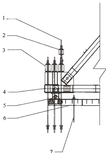
图 2 挂篮锚固系统
