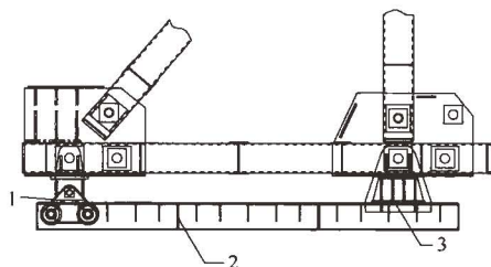
图 4 挂篮行走系统
