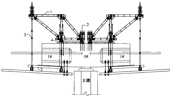
图 1 挂篮系统
