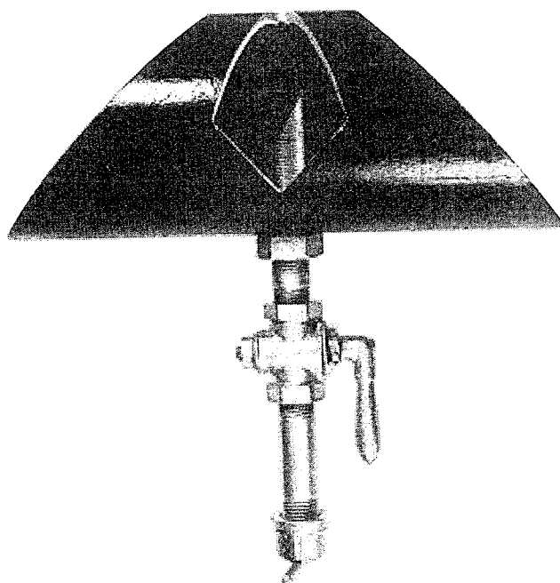
图4 沥青在线取样装置
