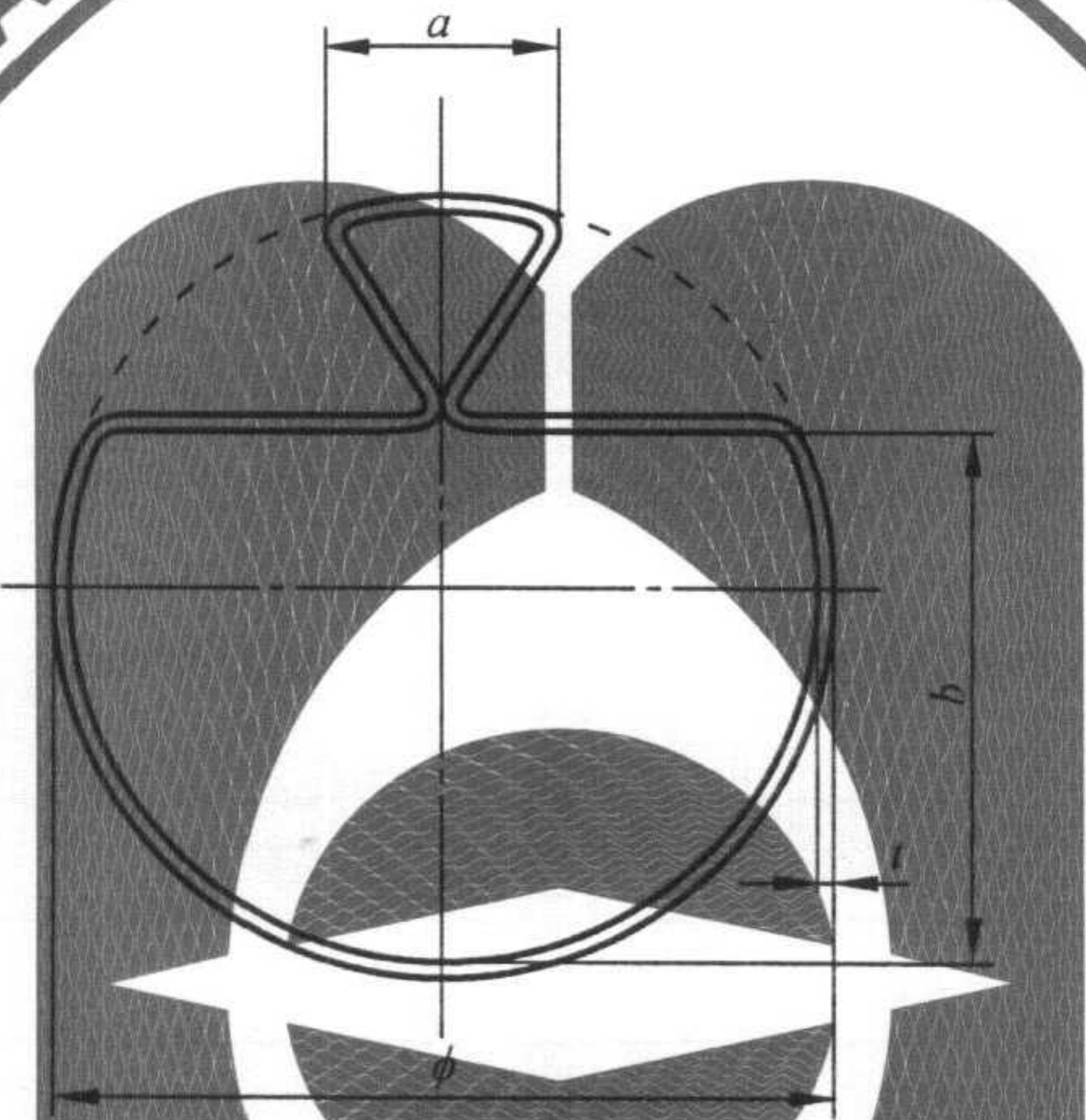
图 3 燕尾柱
